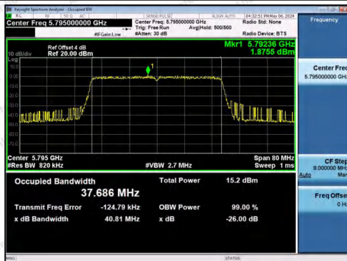
11AX40MIMO-Ant1-5795
