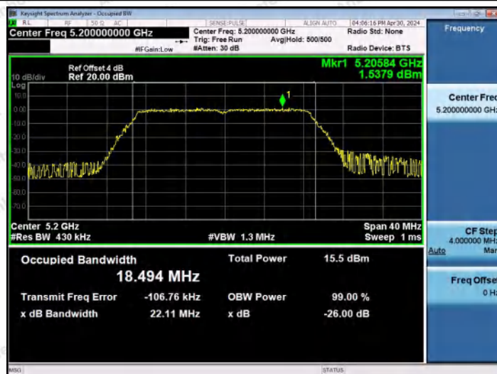
11N20MIMO-Ant1-5200
