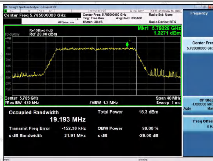
11AX20MIMO-Ant1-5785
