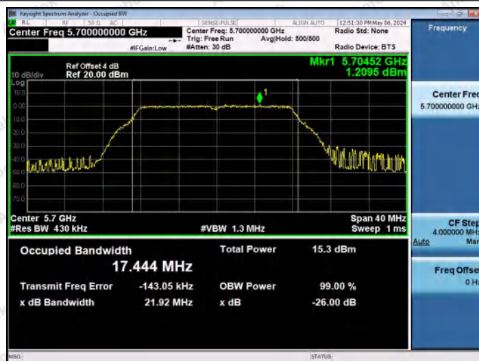
11A-Ant0-5700
