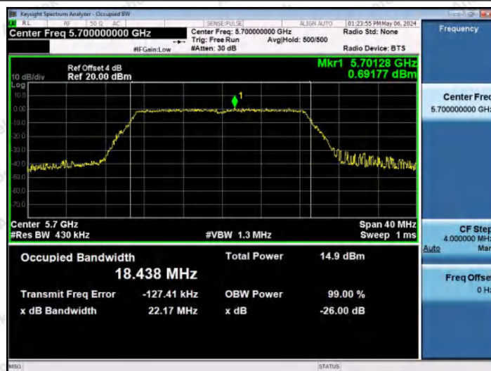
11N20MIMO-Ant0-5700
