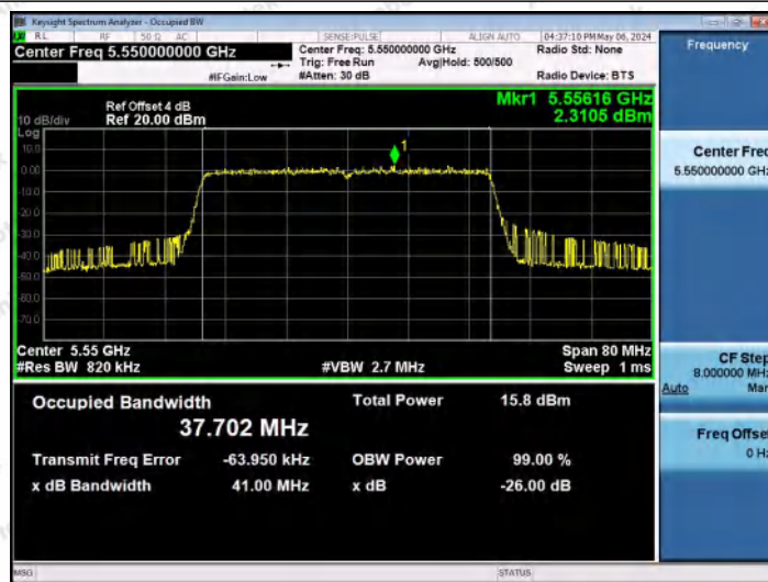
11AX40MIMO-Ant0-5550
