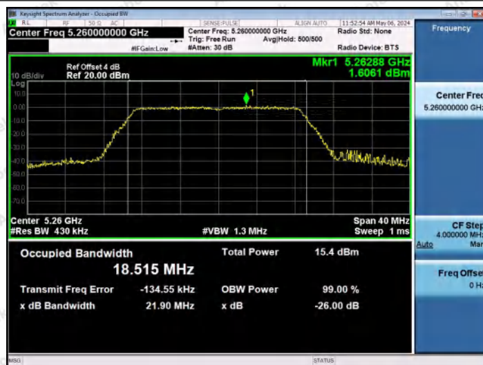
11AC20MIMO-Ant1-5260
