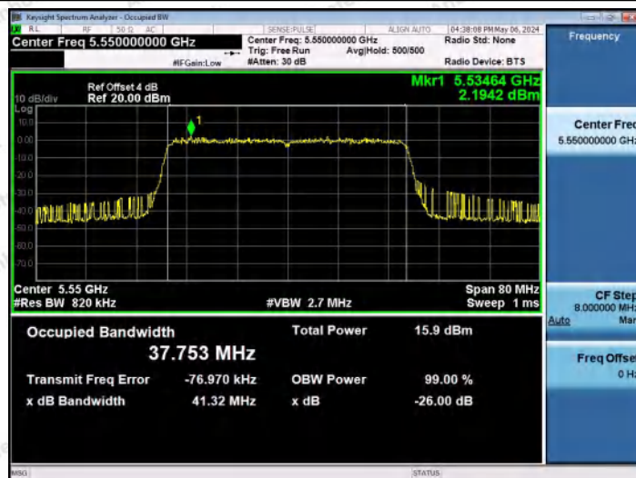
11AX40MIMO-Ant1-5550
