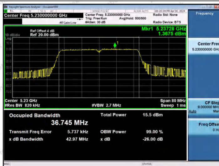
11AC40MIMO-Ant0-5230
