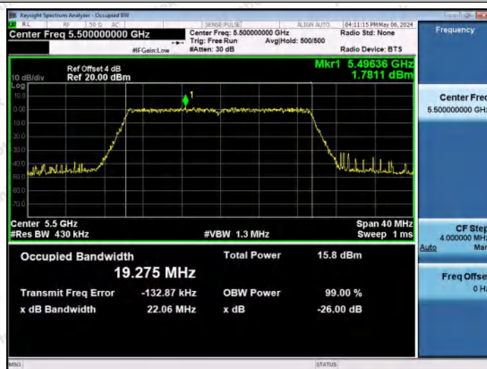
11AX20MIMO-Ant1-5500
