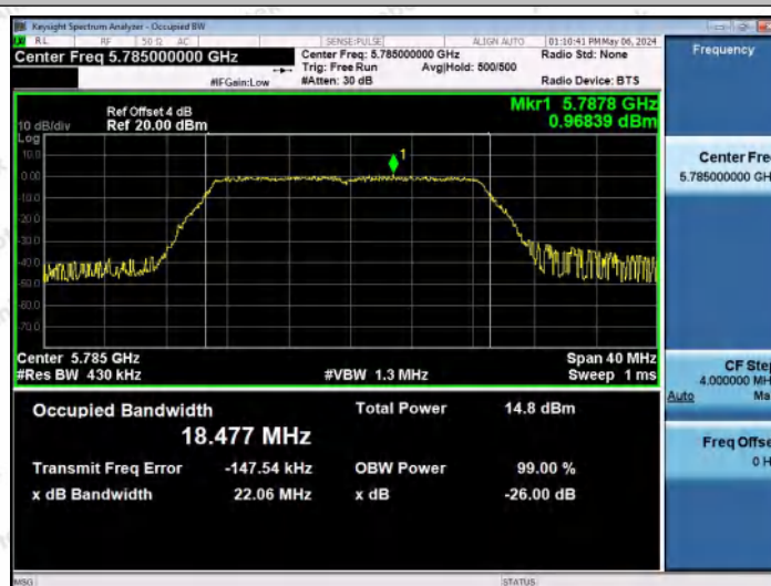
11N20MIMO-Ant0-5785
