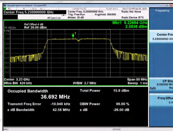
11N40MIMO-Ant0-5230
