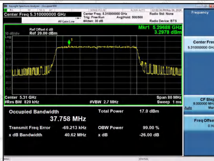
11AX40MIMO-Ant0-5310
