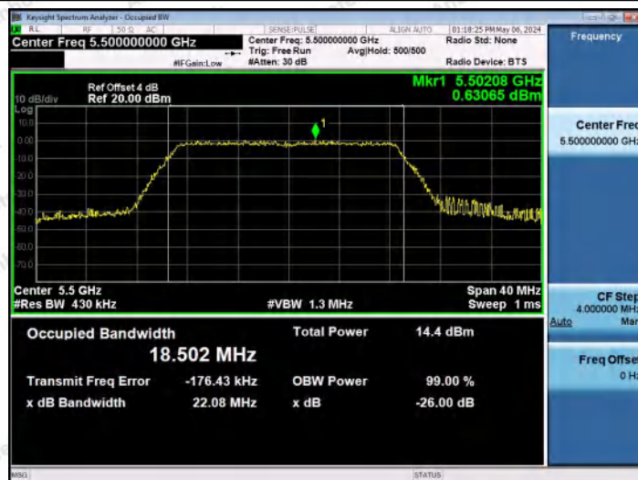
11N20MIMO-Ant0-5500
