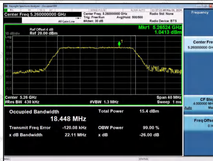
11N20MIMO-Ant1-5260
