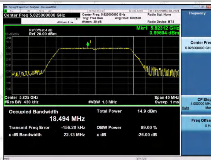
11N20MIMO-Ant0-5825
