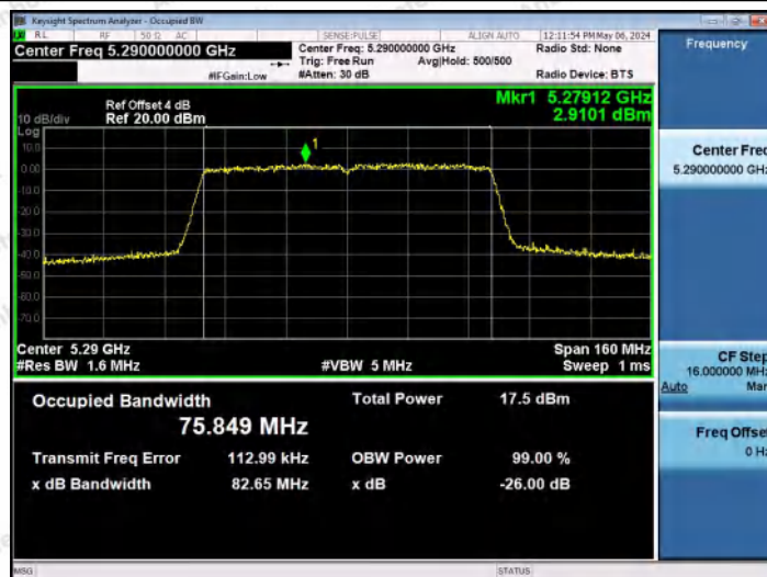
11AC80MIMO-Ant1-5290
