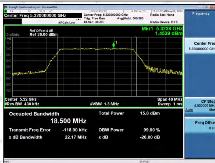
11N20MIMO-Ant0-5320
