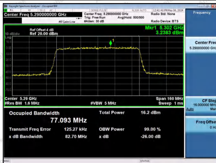
11AX80MIMO-Ant1-5290
