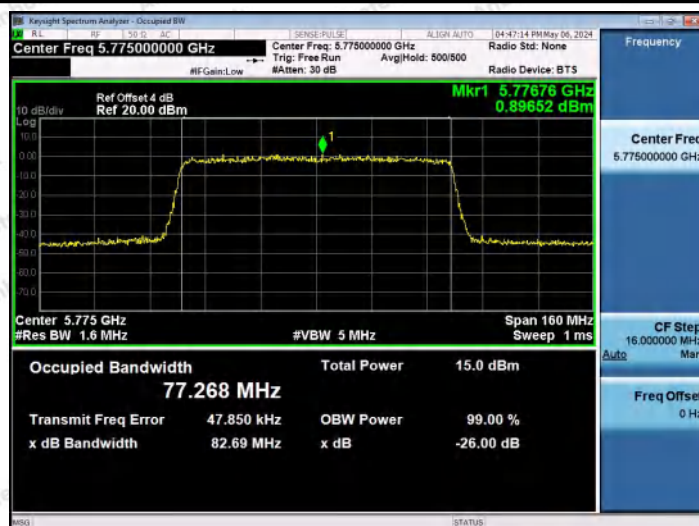
11AX80MIMO-Ant0-5775
