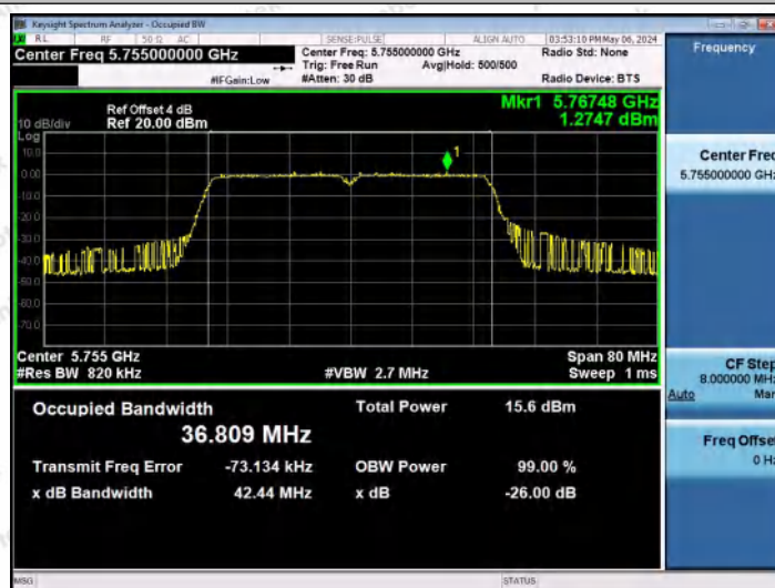
11AC40MIMO-Ant0-5755
