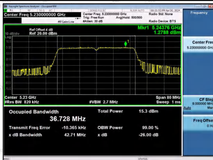
11AC40MIMO-Ant1-5230
