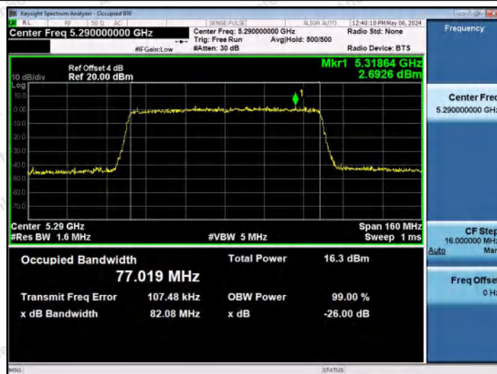
11AX80MIMO-Ant0-5290
