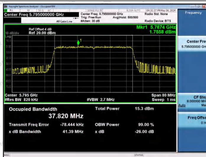
11AX40MIMO-Ant0-5795
