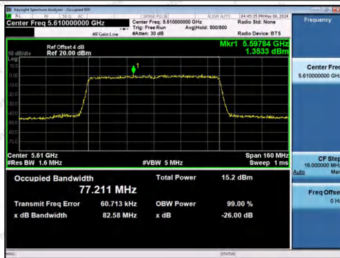
11AX80MIMO-Ant1-5610
