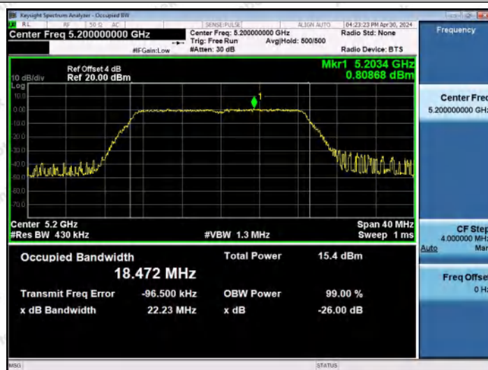
11AC20MIMO-Ant0-5200
