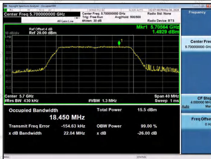
11AC20MIMO-Ant0-5700
