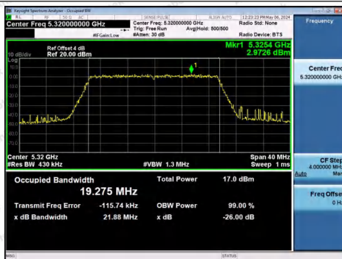
11AX20MIMO-Ant0-5320
