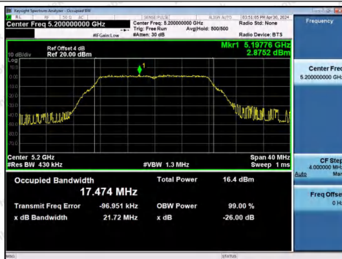
11A-Ant0-5200
