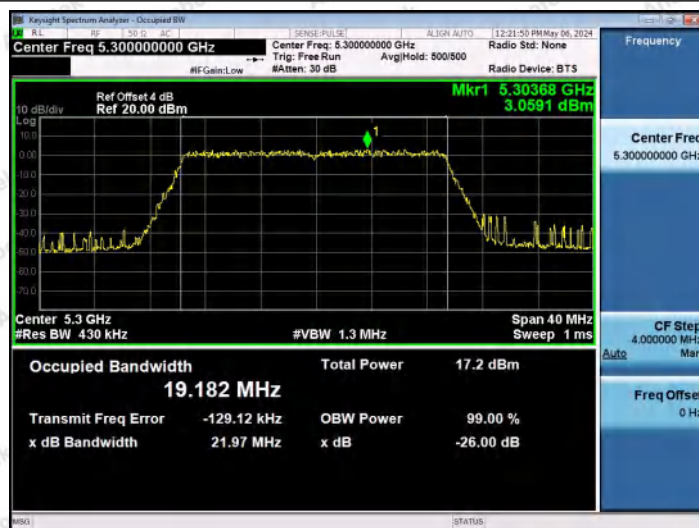
11AX20MIMO-Ant1-5300
