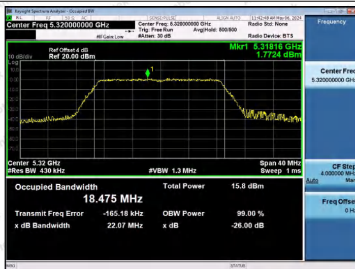
11N20MIMO-Ant1-5320
