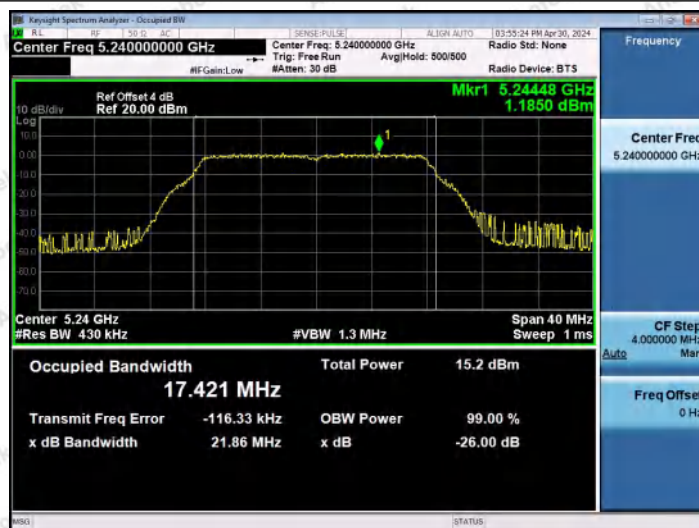
11A-Ant0-5240
