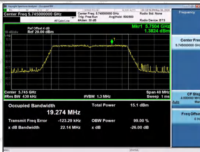
11AX20MIMO-Ant1-5745
