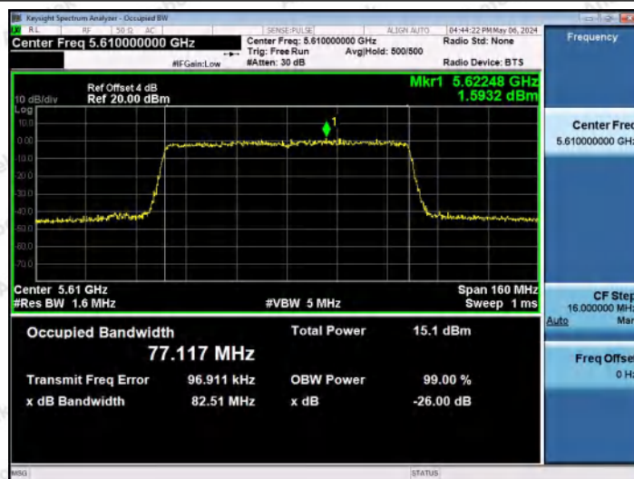
11AX80MIMO-Ant0-5610
