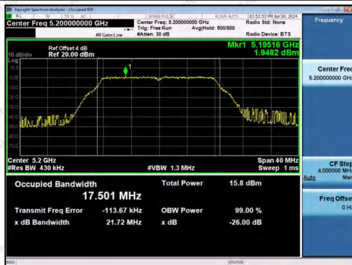
11A-Ant1-5200
