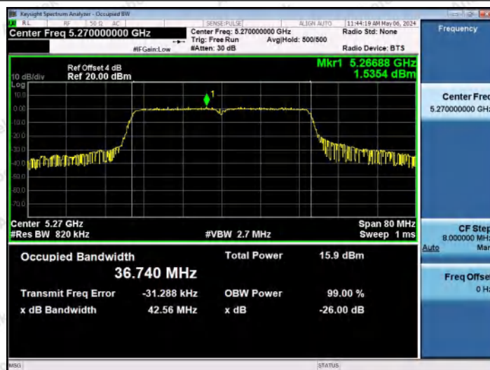
11N40MIMO-Ant0-5270
