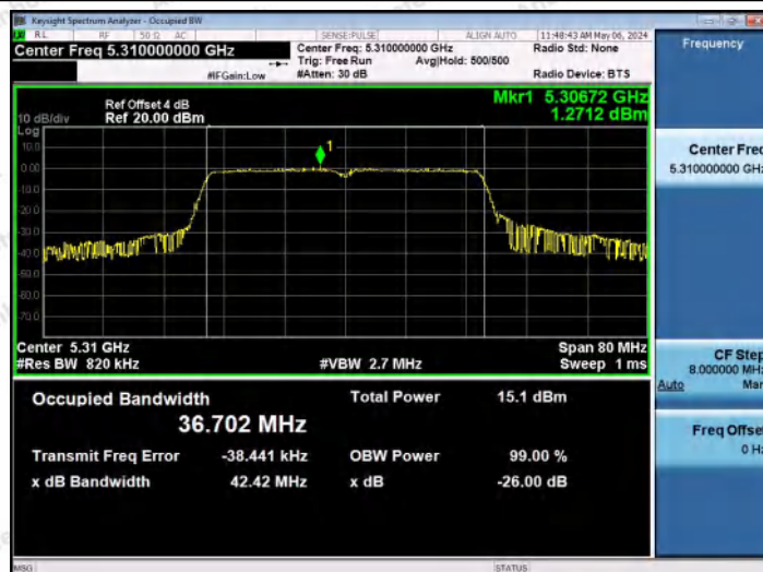
11N40MIMO-Ant0-5310
