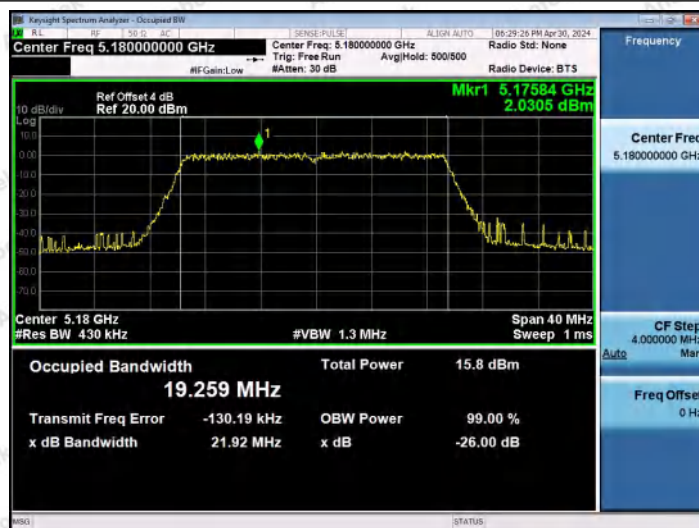
11AX20MIMO-Ant0-5180
