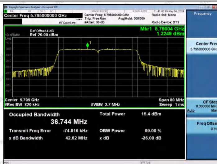
11N40MIMO-Ant0-5795
