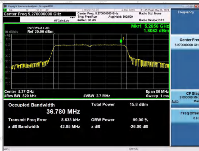
11N40MIMO-Ant1-5270
