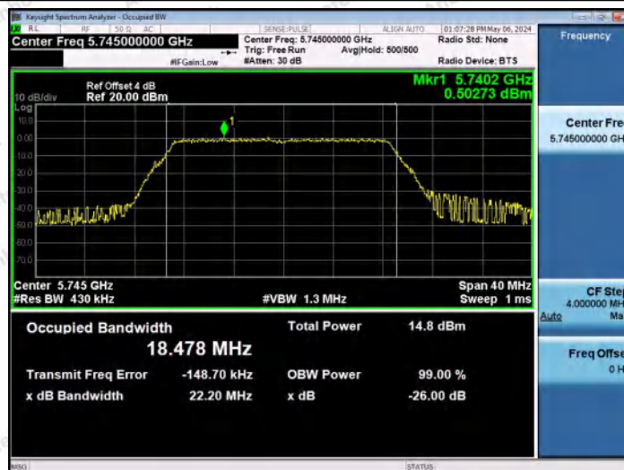
11N20MIMO-Ant0-5745
