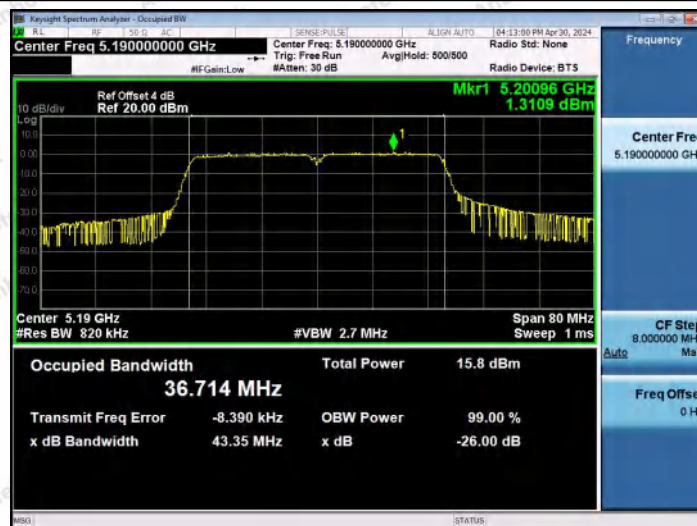
11N40MIMO-Ant0-5190
