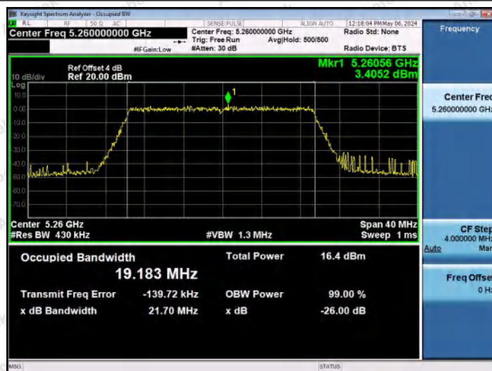
11AX20MIMO-Ant0-5260
