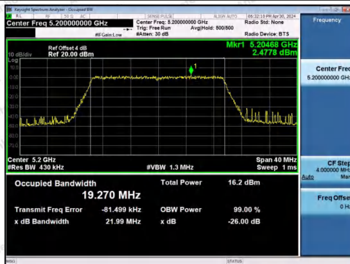
11AX20MIMO-Ant0-5200
