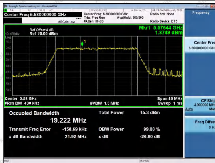
11AX20MIMO-Ant1-5580
