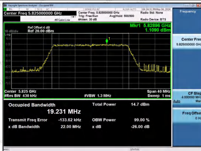
11AX20MIMO-Ant1-5825
