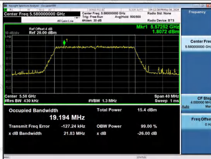
11AX20MIMO-Ant0-5580
