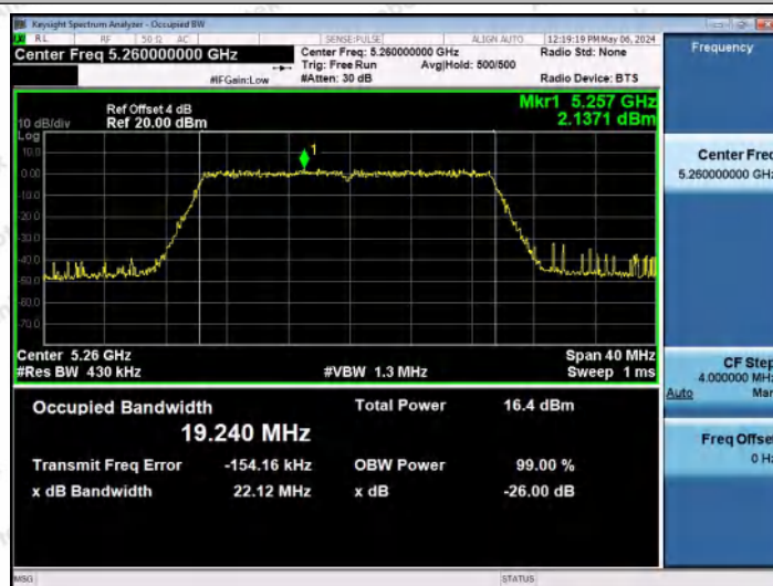
11AX20MIMO-Ant1-5260
