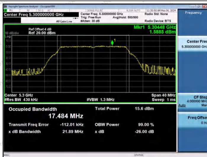
11A-Ant0-5300
