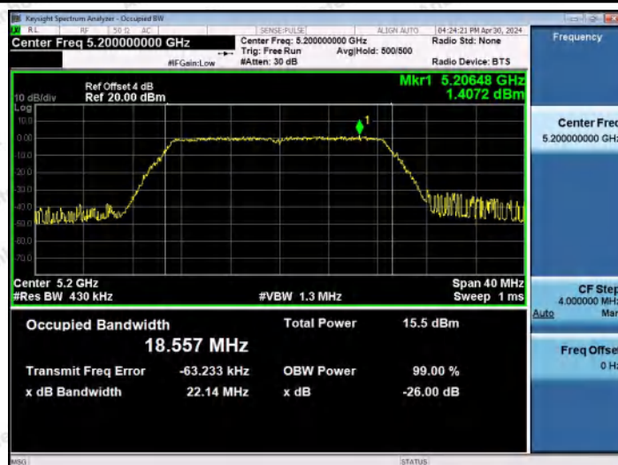
11AC20MIMO-Ant1-5200
