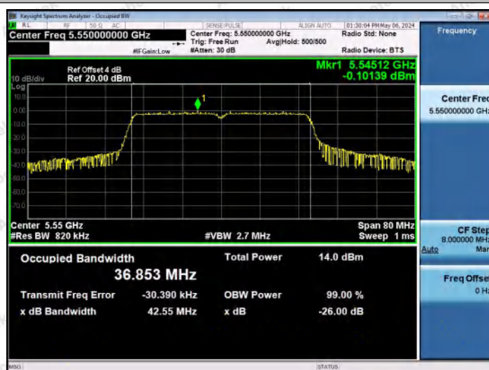
11N40MIMO-Ant0-5550
