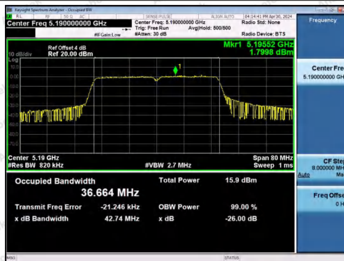
11N40MIMO-Ant1-5190
