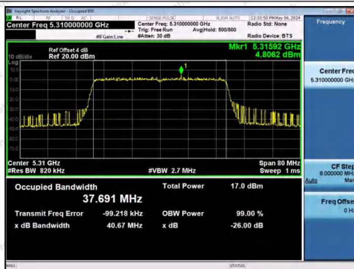
11AX40MIMO-Ant1-5310
