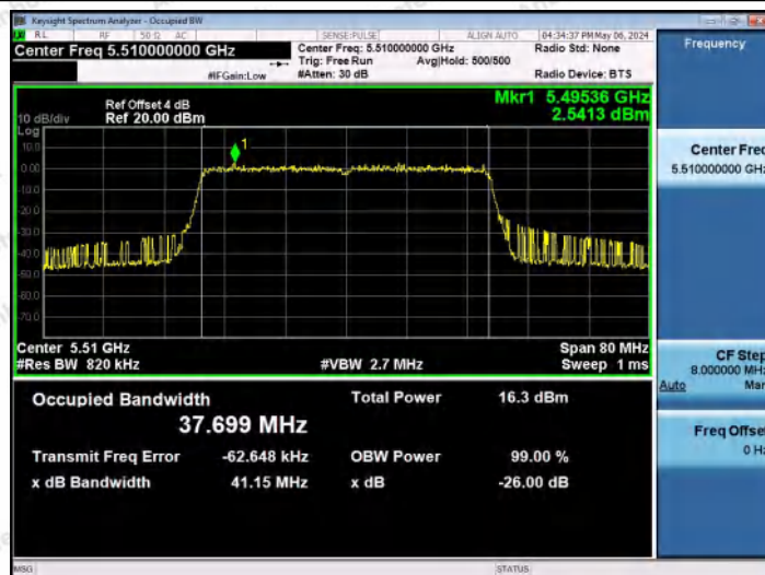
11AX40MIMO-Ant0-5510
