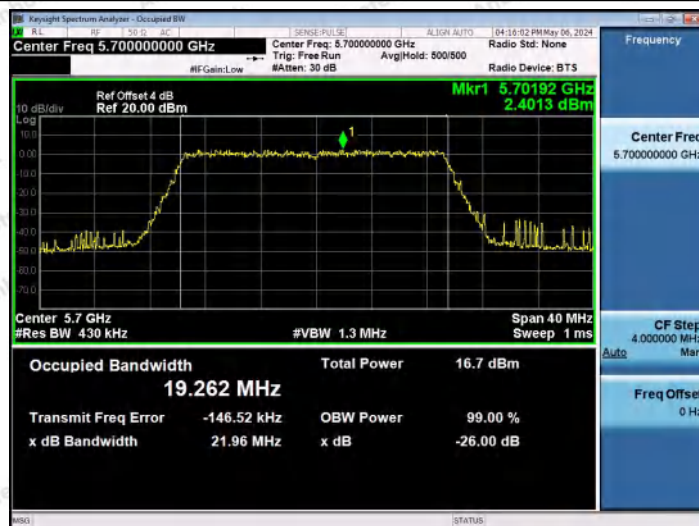
11AX20MIMO-Ant1-5700
