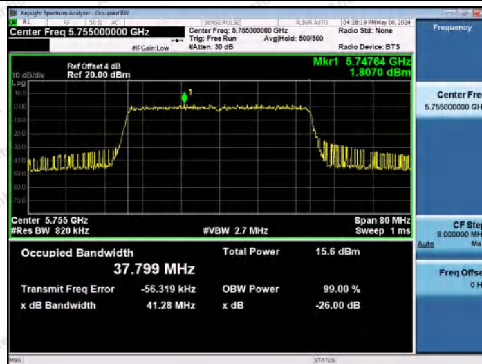
11AX40MIMO-Ant0-5755
