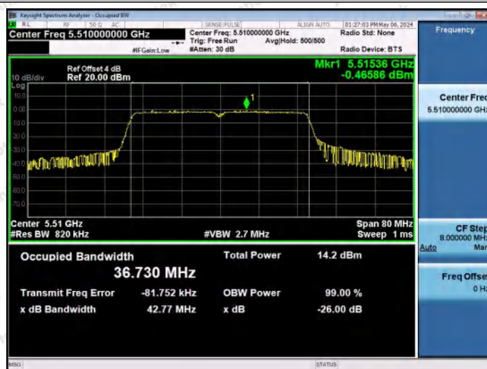
11N40MIMO-Ant0-5510
