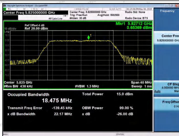
11N20MIMO-Ant1-5825
