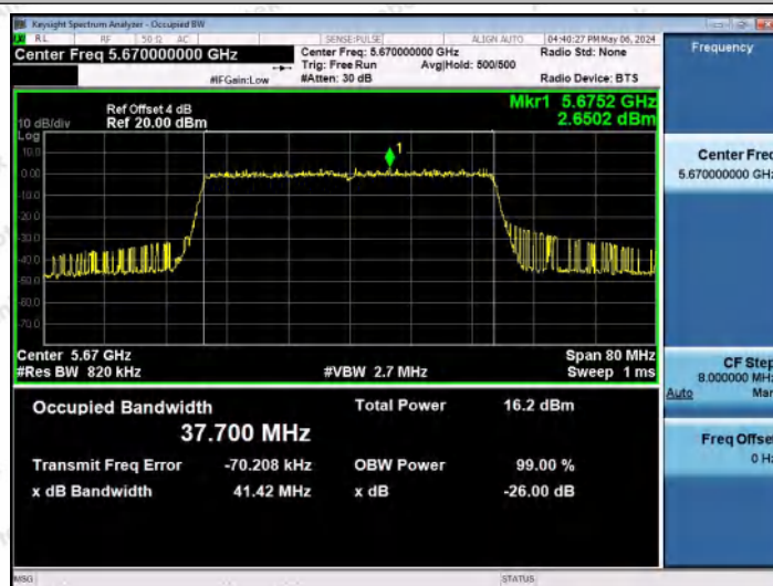
11AX40MIMO-Ant1-5670
