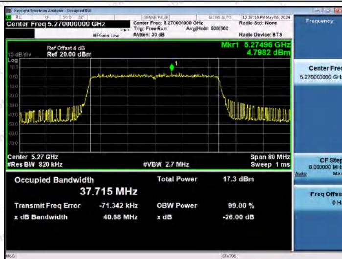
11AX40MIMO-Ant0-5270
