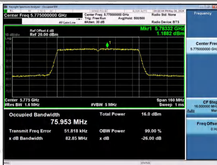
11AC80MIMO-Ant0-5775
