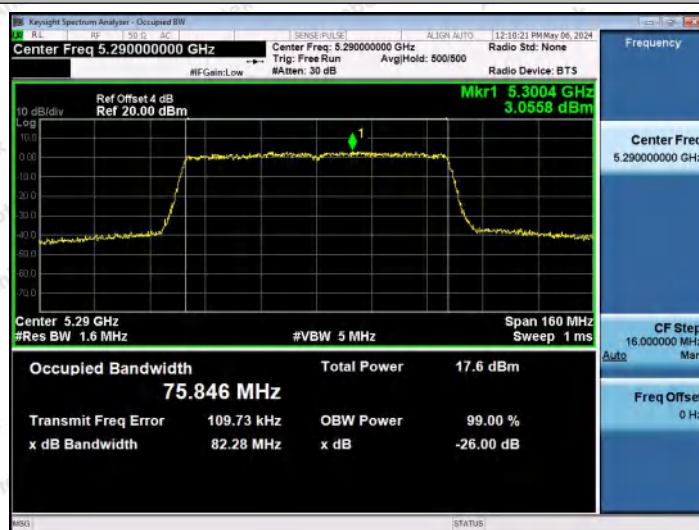
11AC80MIMO-Ant0-5290
