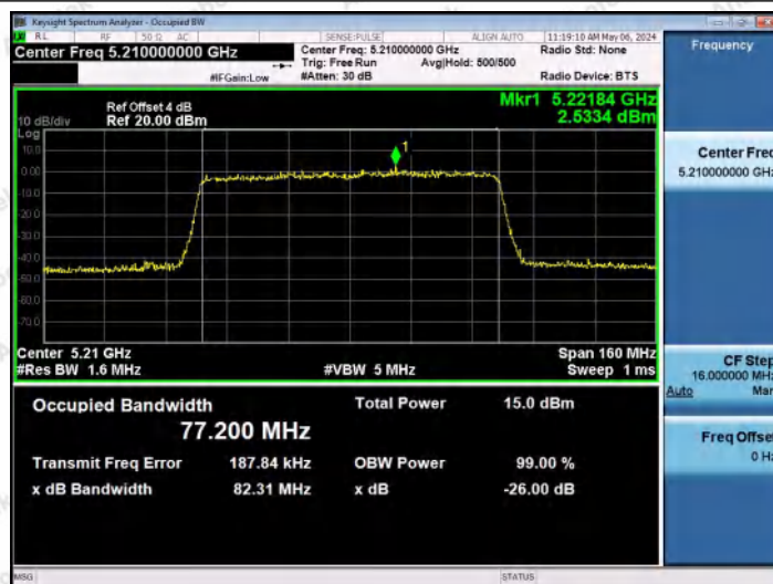
11AX80MIMO-Ant0-5210
