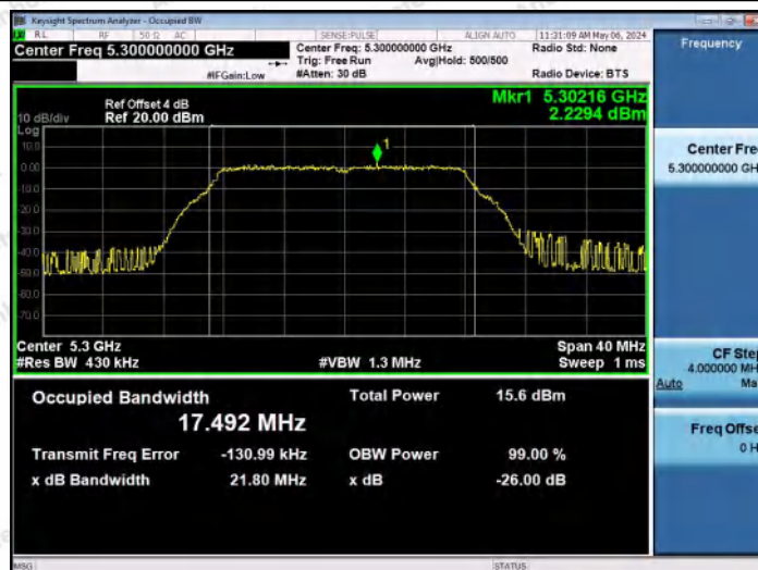
11A-Ant1-5300
