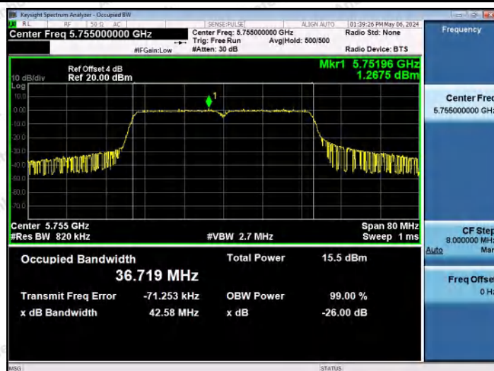
11N40MIMO-Ant1-5755
