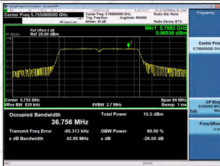
11N40MIMO-Ant0-5755
