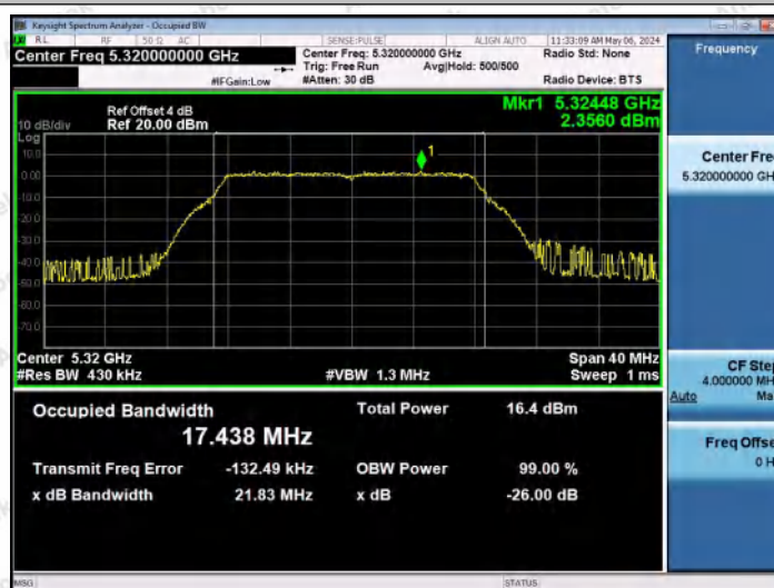
11A-Ant0-5320
