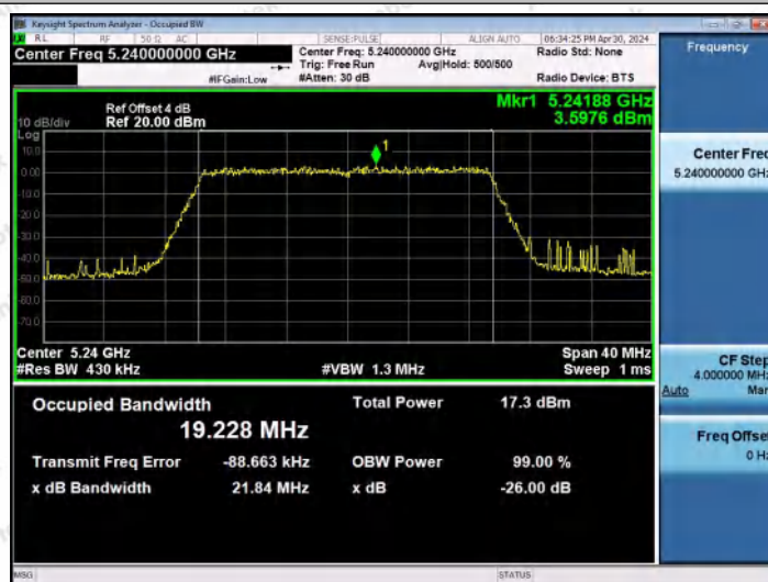
11AX20MIMO-Ant0-5240
