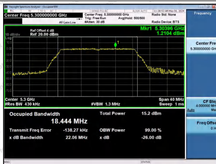
11N20MIMO-Ant0-5300
