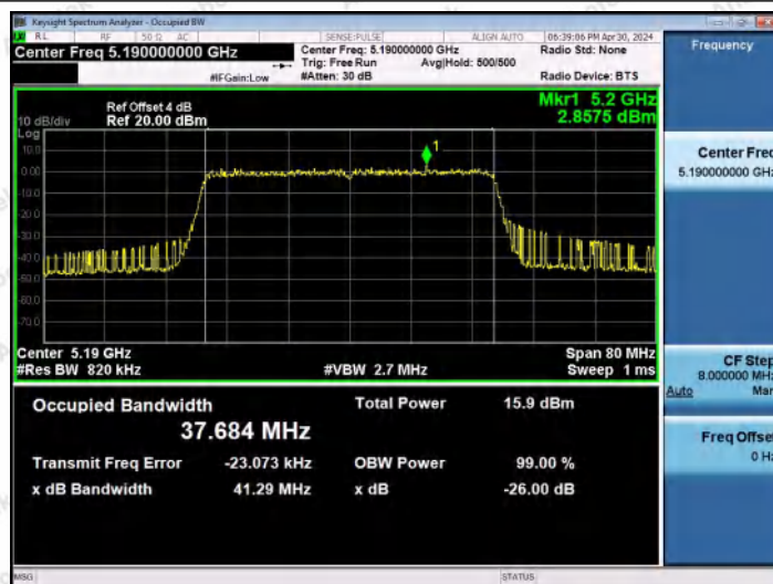
11AX40MIMO-Ant0-5190
