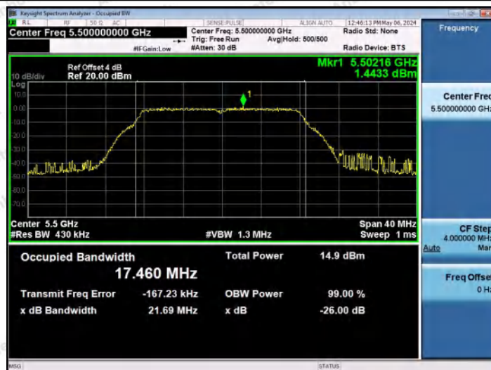
11A-Ant0-5500
