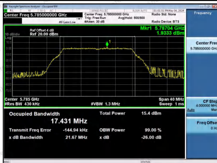
11A-Ant0-5785
