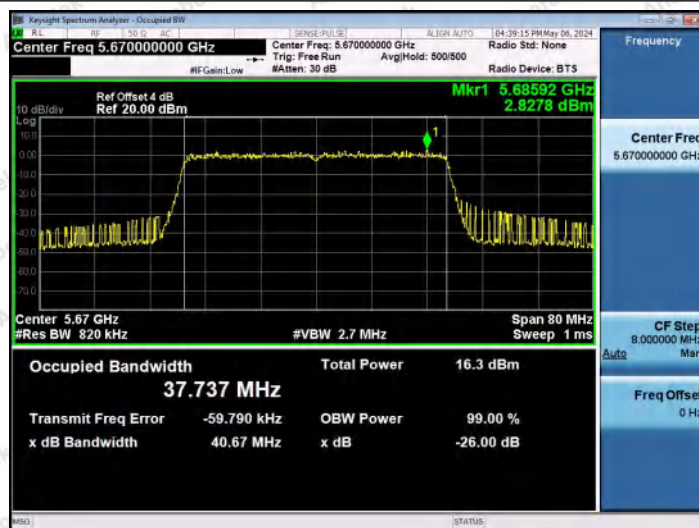
11AX40MIMO-Ant0-5670
