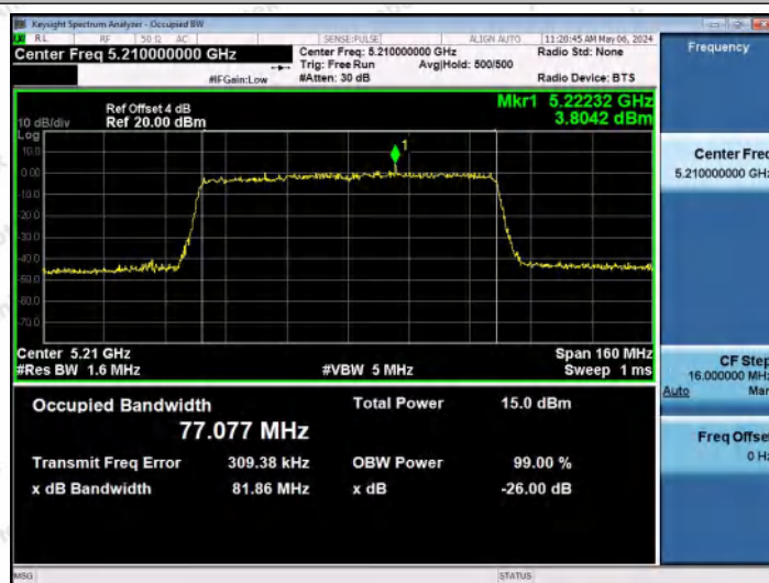
11AX80MIMO-Ant1-5210
