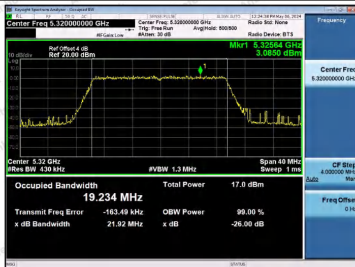
11AX20MIMO-Ant1-5320
