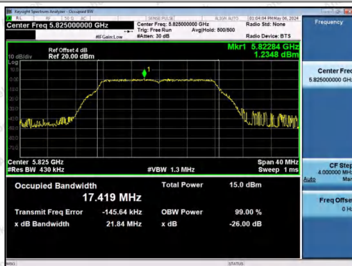
11A-Ant0-5825
