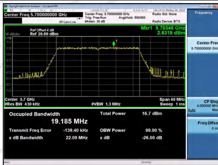
11AX20MIMO-Ant0-5700
