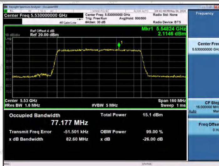
11AX80MIMO-Ant0-5530
