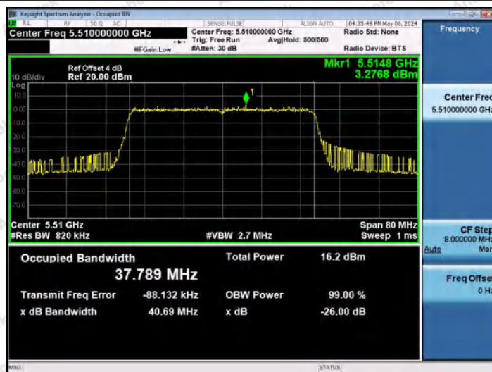
11AX40MIMO-Ant1-5510
