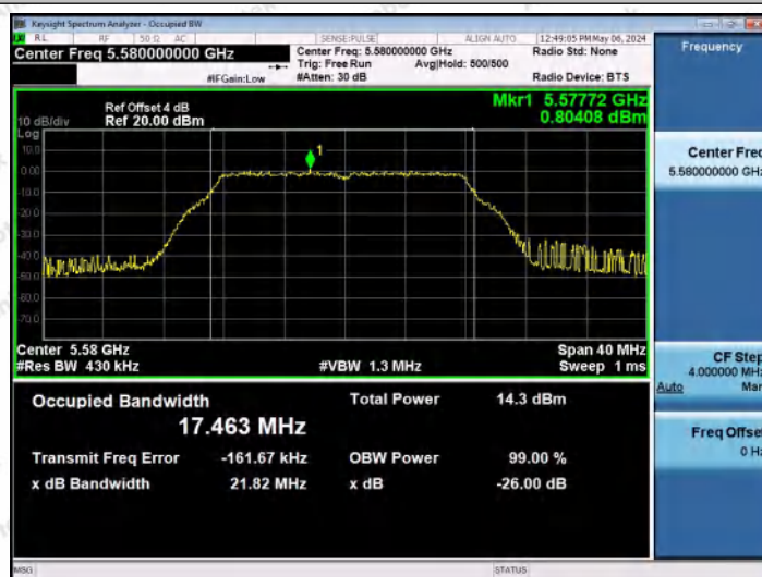
11A-Ant0-5580
