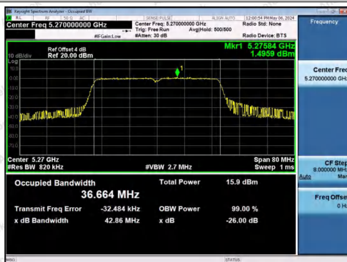
11AC40MIMO-Ant0-5270
