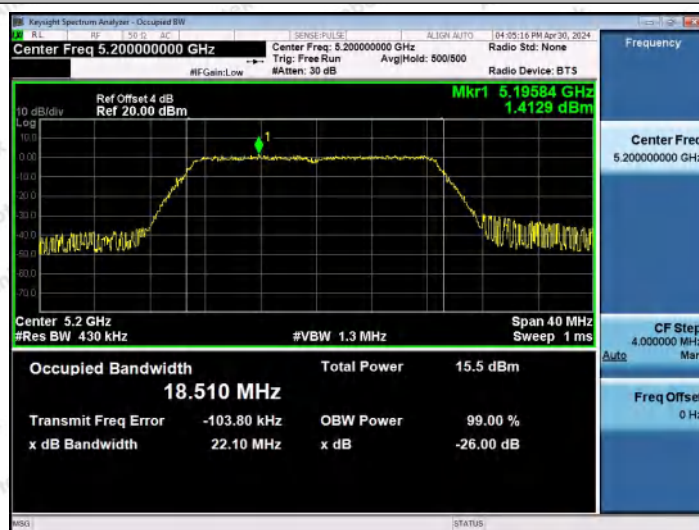
11N20MIMO-Ant0-5200
