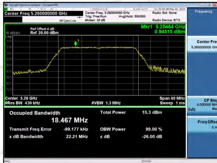
11N20MIMO-Ant0-5260
