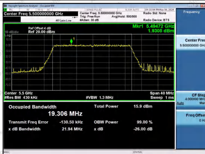
11AX20MIMO-Ant0-5500
