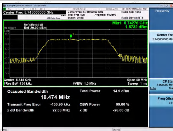
11N20MIMO-Ant1-5745
