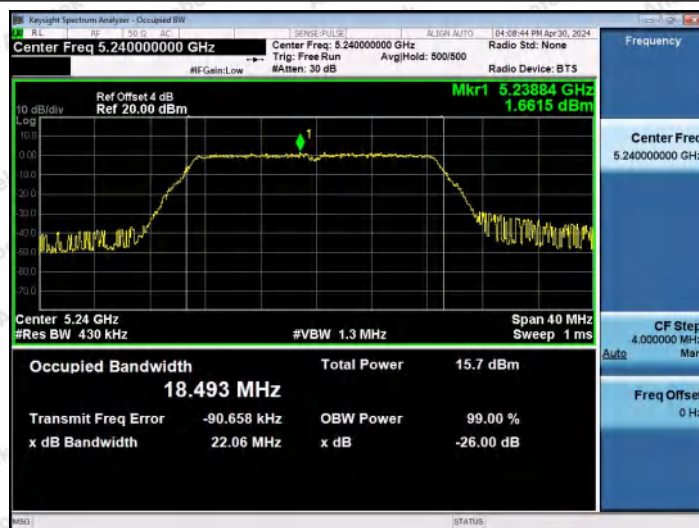
11N20MIMO-Ant0-5240
