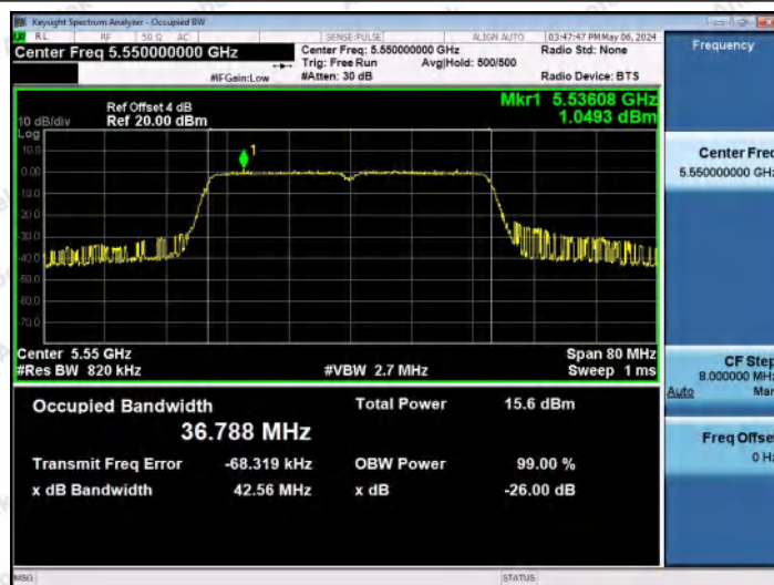
11AC40MIMO-Ant0-5550
