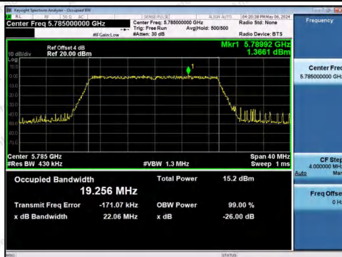
11AX20MIMO-Ant0-5785
