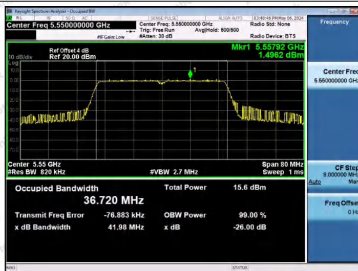
11AC40MIMO-Ant1-5550
