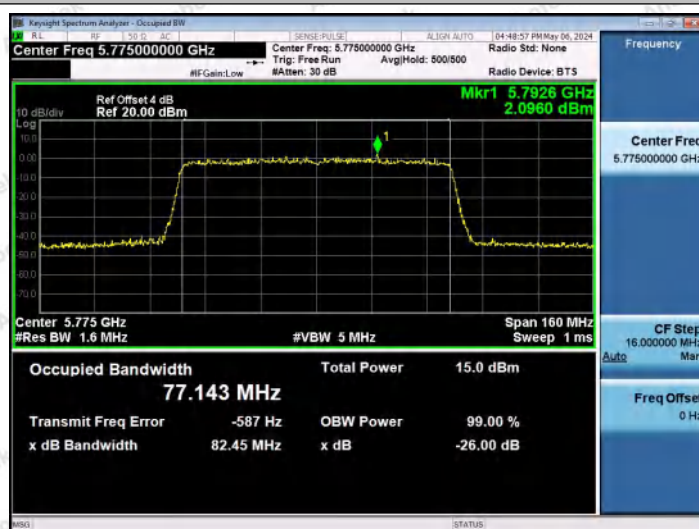
11AX80MIMO-Ant1-5775
