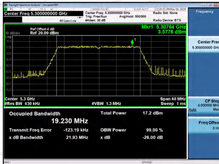
11AX20MIMO-Ant0-5300
