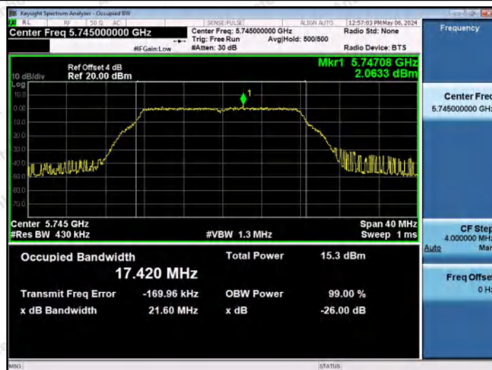
11A-Ant0-5745
