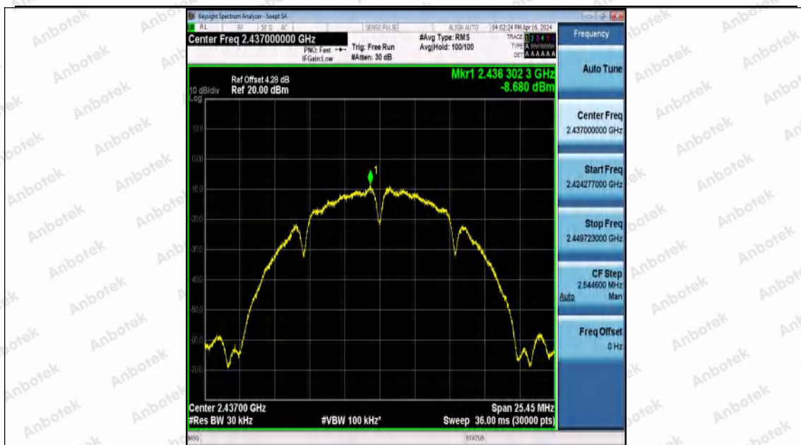
11B-Ant0-2437-PASS
