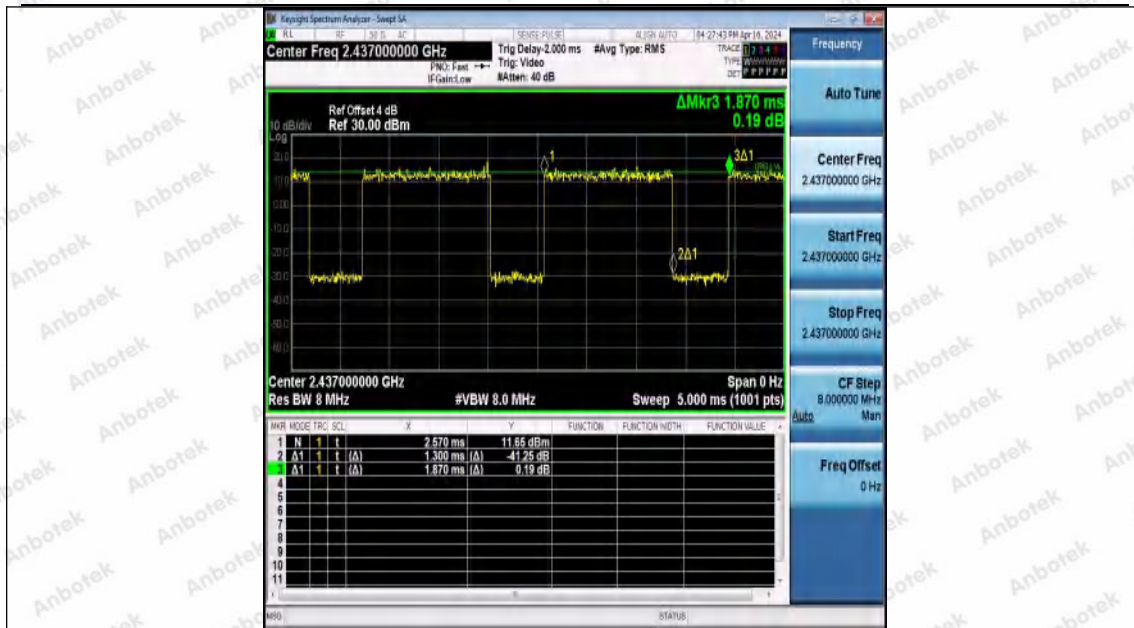
NTNV-11N20MIMO-Ant0-2437
