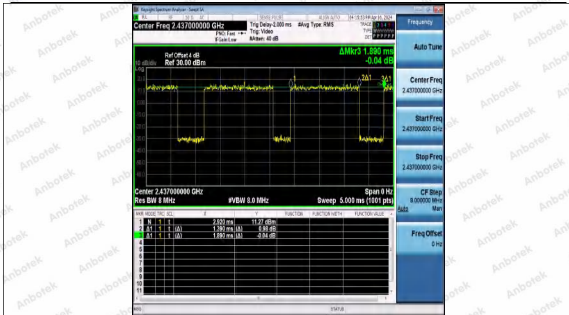
NTNV-11G-Ant0-2437
