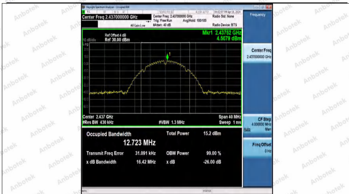
11B-Ant0-2437
