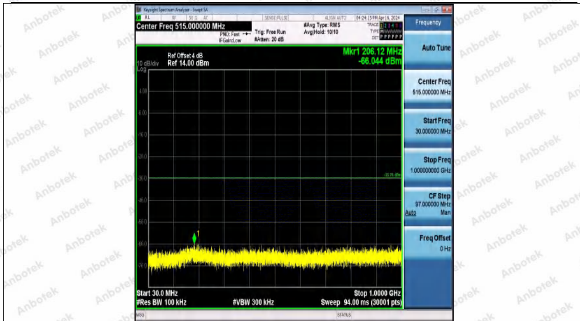
11N20MIMO-Ant0-2412-30~1000-PASS
