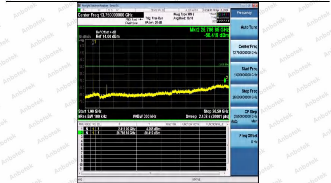
11B-Ant0-2412-1000~26500-PASS
