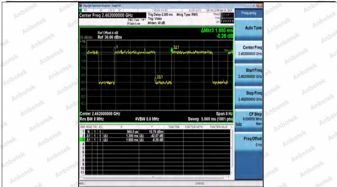
NTNV-11G-Ant0-2462
