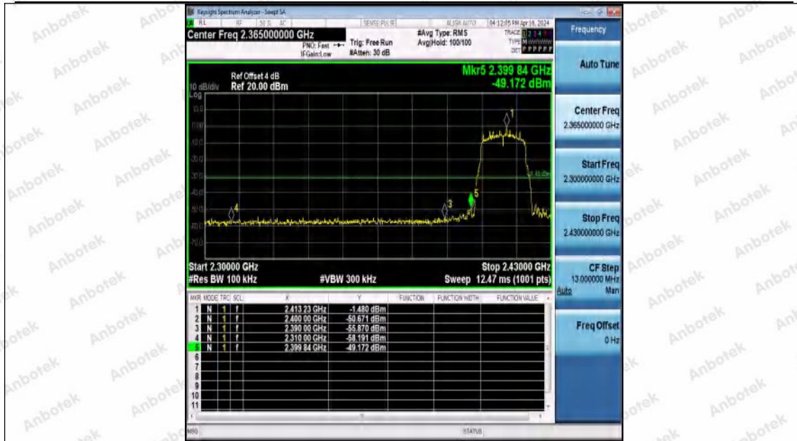
11G-Ant0-2412-PASS
