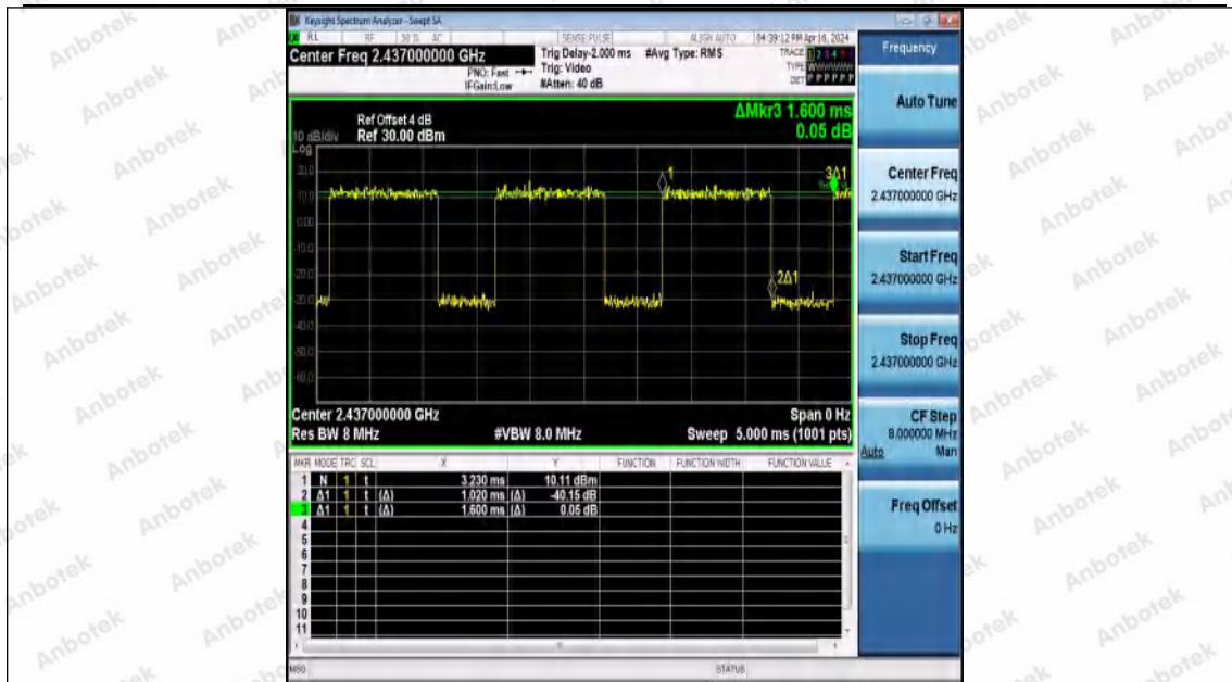
NTNV-11AX20MIMO-Ant0-2437
