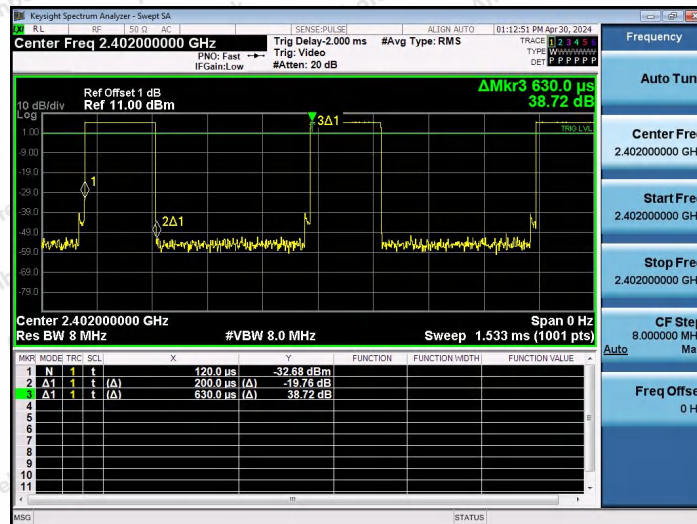
NTNV-BLE_2M-Ant0-2402
