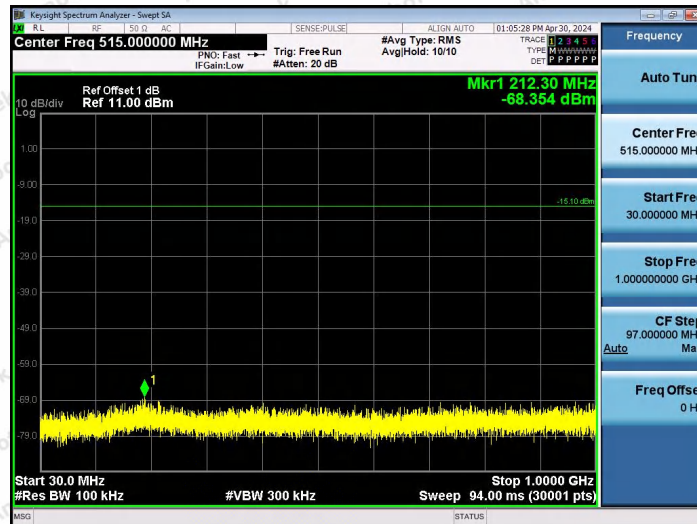
BLE_1M-Ant0-2402-30~1000-PASS
