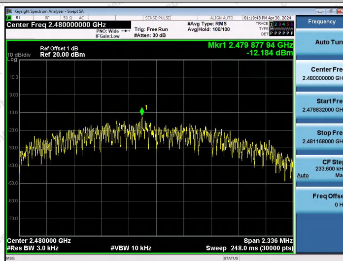
BLE_2M-Ant0-2480-PASS
