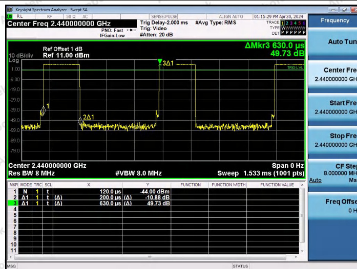
NTNV-BLE_2M-Ant0-2440
