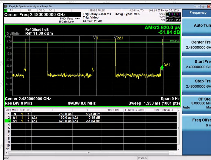
NTNV-BLE_2M-Ant0-2480
