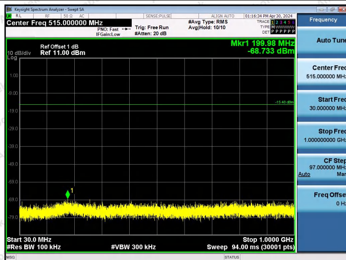
BLE_2M-Ant0-2440-30~1000-PASS
