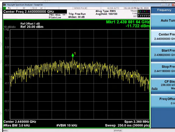
BLE_2M-Ant0-2440-PASS
