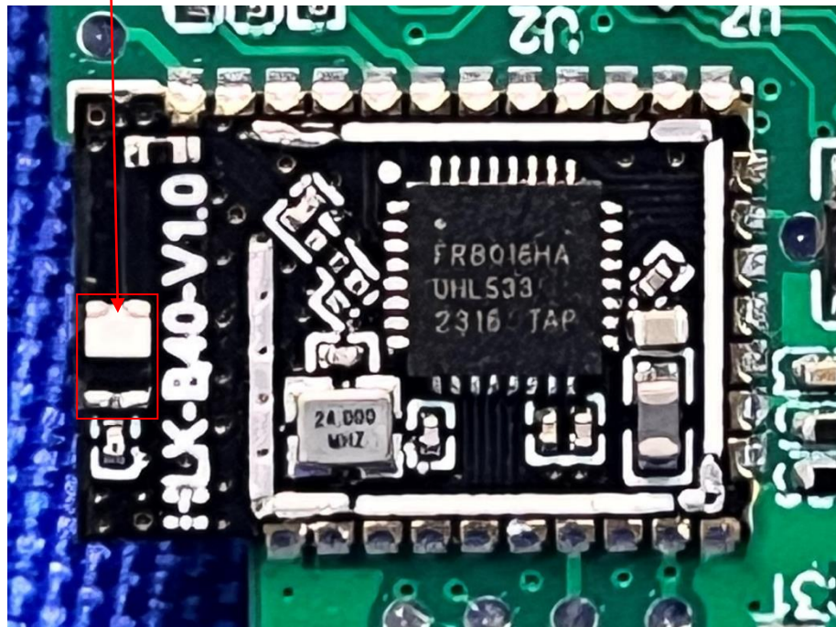
BLE Antenna
