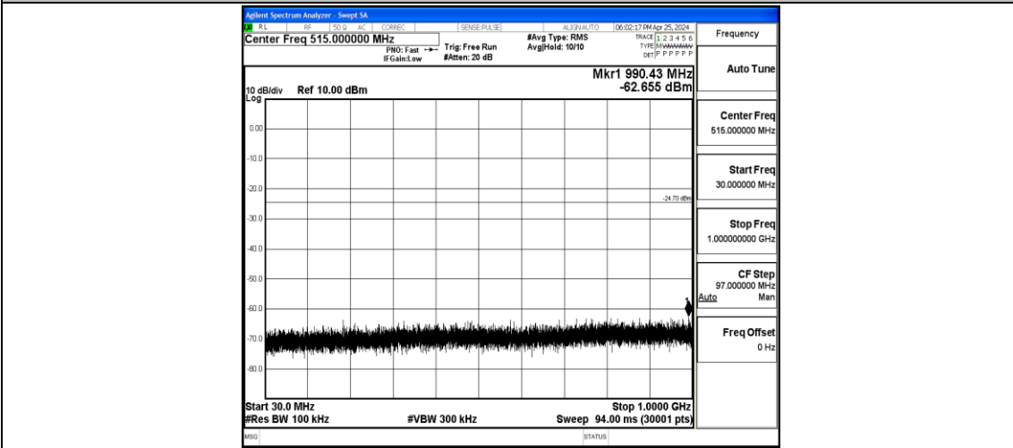
11G-Ant1-2462-30~1000-PASS
