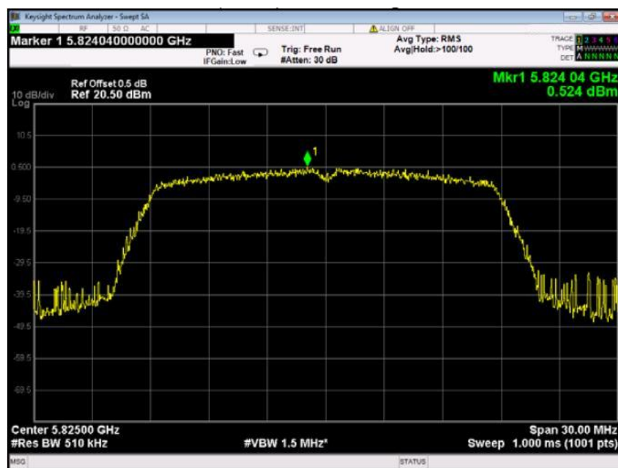
U-NII-3 802.11n(HT20) High CH
