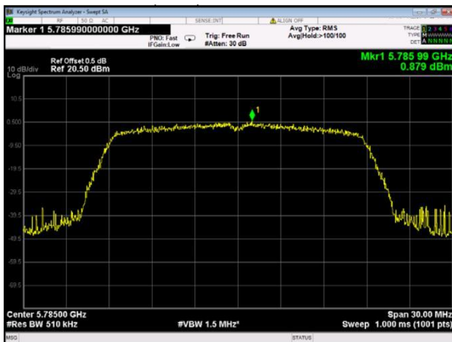
U-NII-3 802.11n(HT20) Middle CH
