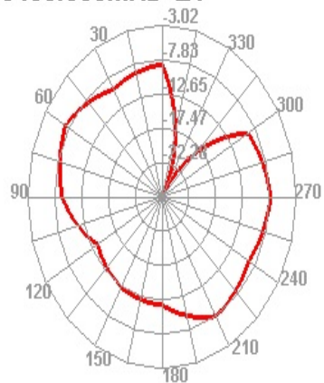
5400.000MHz E1
