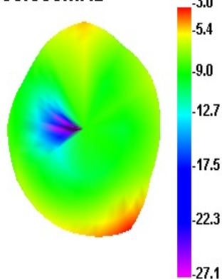
5400.000MHz
