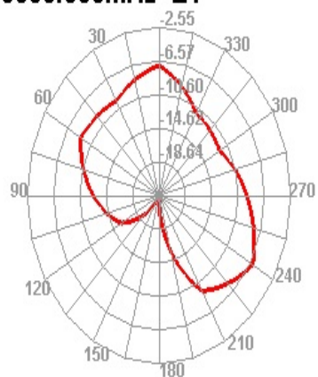
5050.000MHz E1
