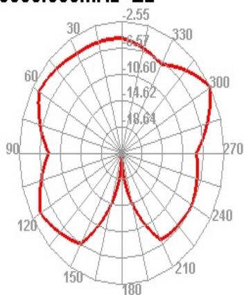
5050.000MHz E2
