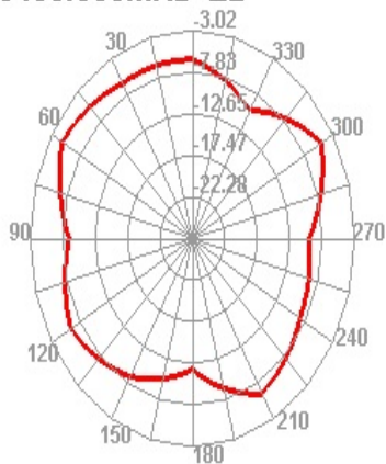
5400.000MHz E2
