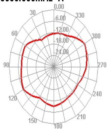
5050.000MHz H
