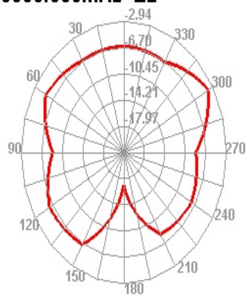
5000.000MHz E2
