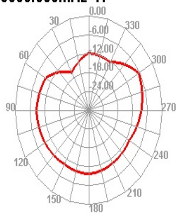
5000.000MHz H
