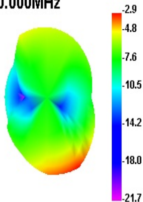
5000.000MHz
