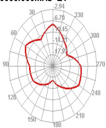
5000.000MHz E1
