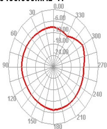
5400.000MHz H
