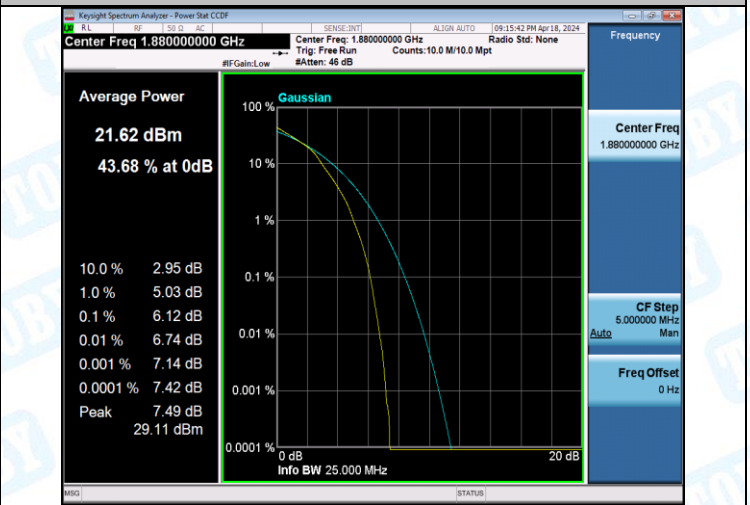
Band2-20MHz-16QAM-19100-27RB#0-PASS
