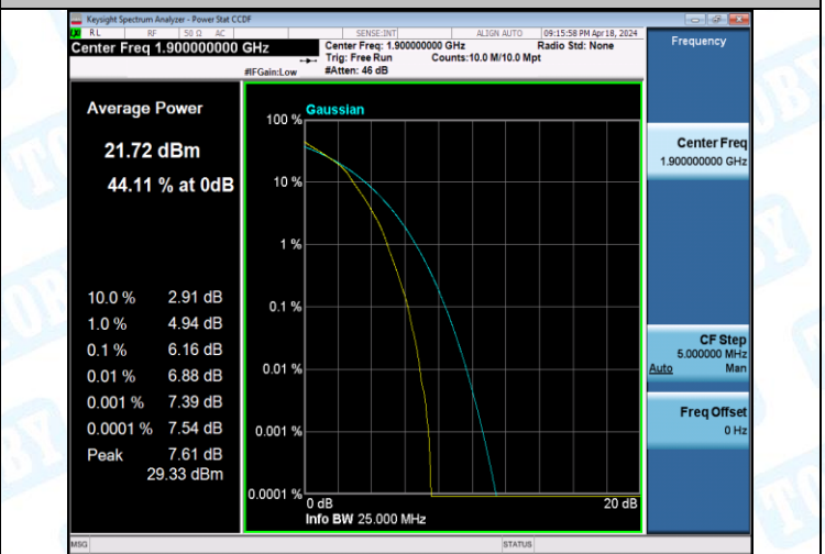
Band2-20MHz-16QAM-19000-27RB#0-PASS
