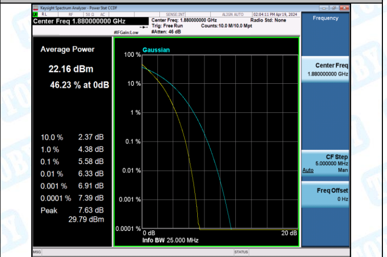
Band2-20MHz-QPSK-19100-100RB#0-PASS
