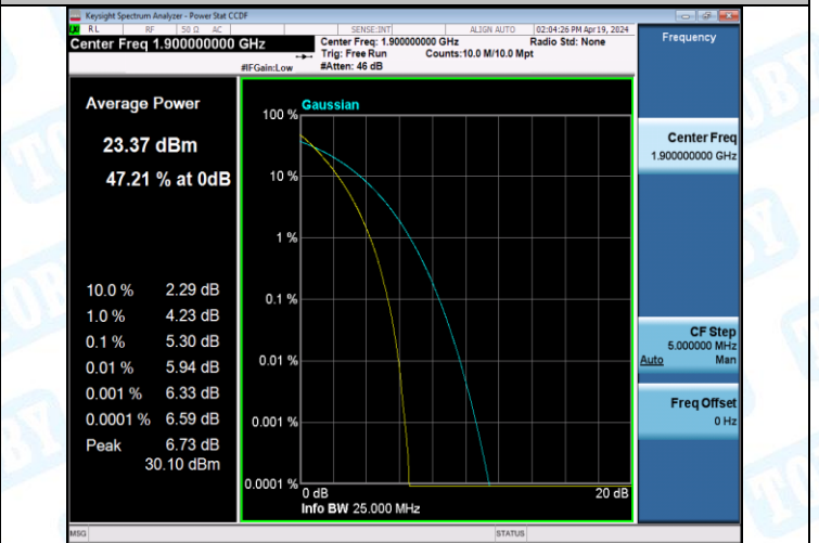
Band2-20MHz-16QAM-18700-27RB#0-PASS
