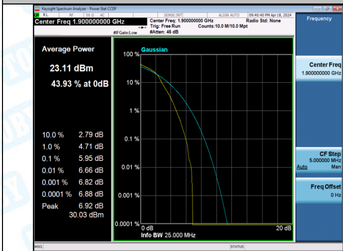
Band2-20MHz-16QAM-19000-1RB#0-PASS
