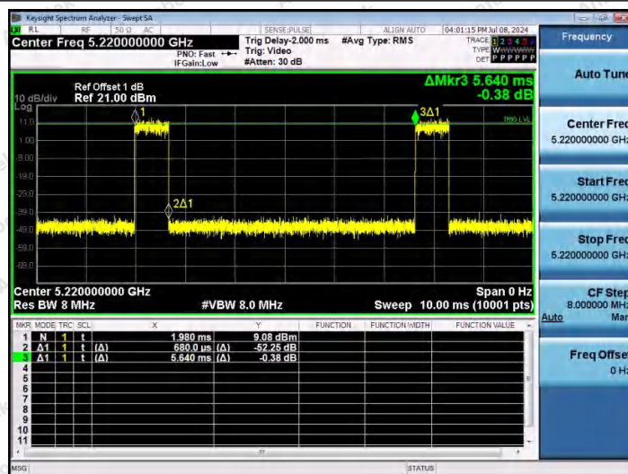
NTNV-11N20SISO-Ant1-5220
