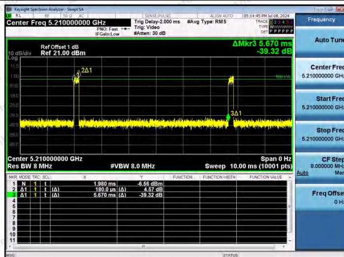
NTNV-11AC80SISO-Ant1-5210
