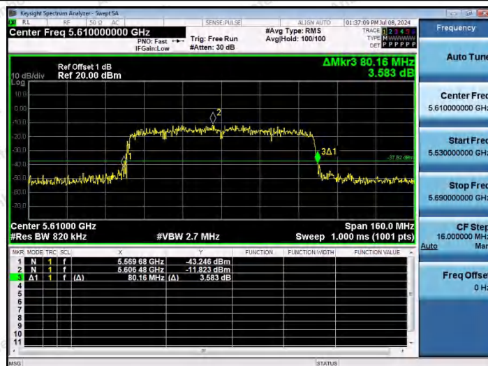
11AC80SISO-Ant1-5610
