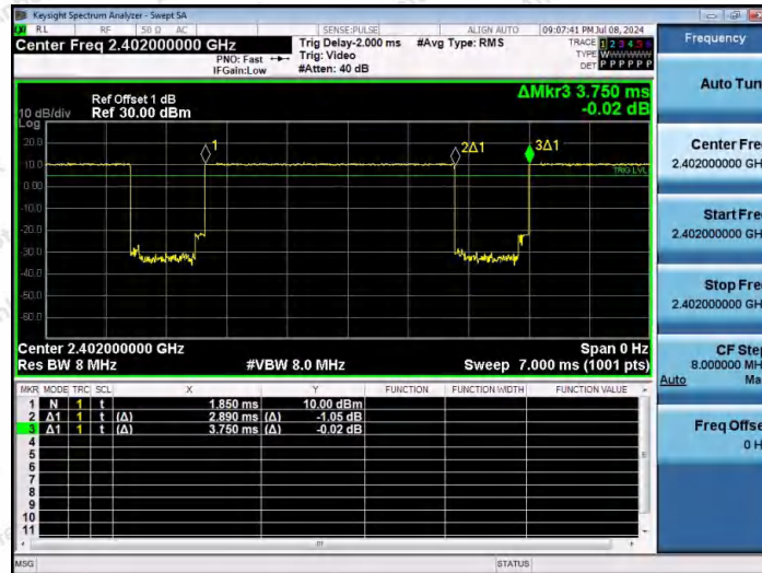
NTNV-2DH5-Ant1-2402
