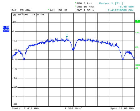
b_2412MHz
