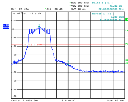
g_2462MHz
