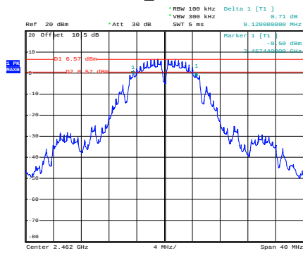
b_2462MHz
