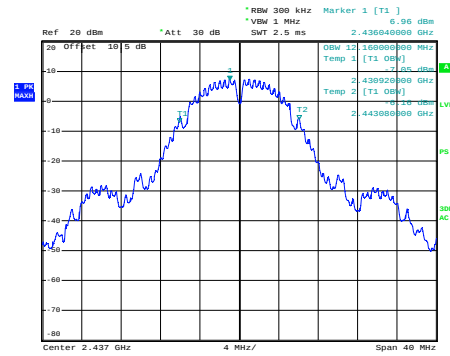
b_2437MHz
