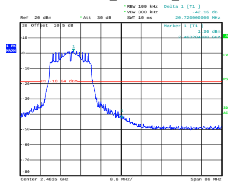
n20_2462MHz
