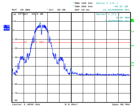
b_2462MHz
