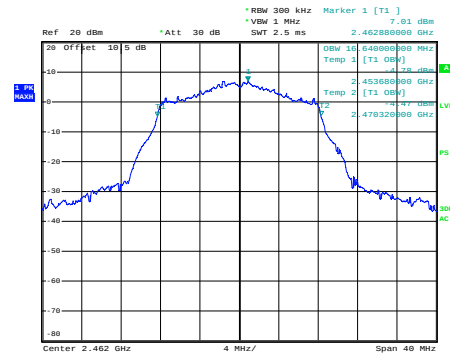
g_2462MHz
