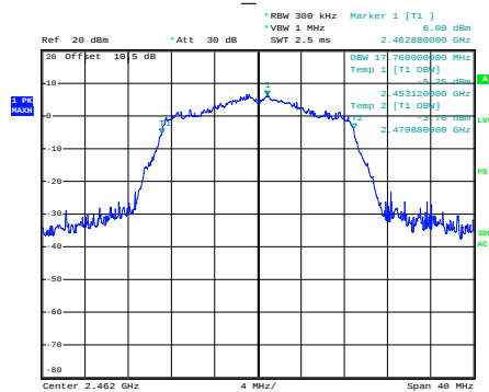
n20_2462MHz
