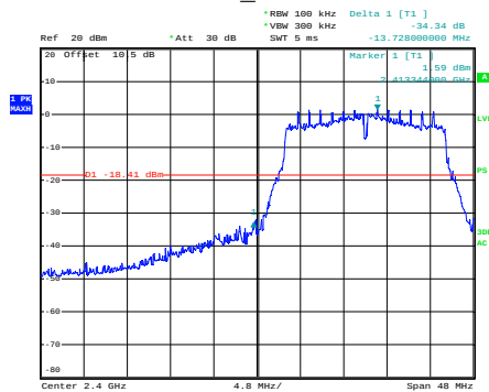
n20_2412MHz
