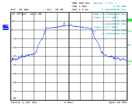
g_2437MHz
