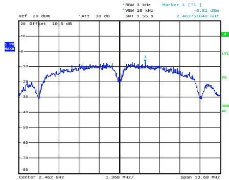
b_2462MHz
