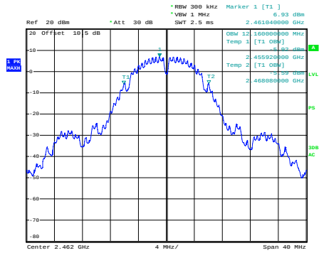
b_2462MHz
