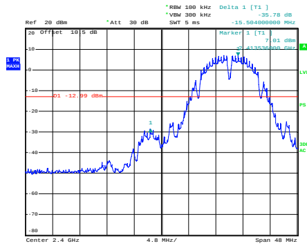
b_2412MHz
