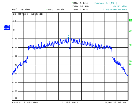
g_2462MHz
