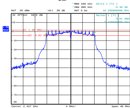
g_2437MHz
