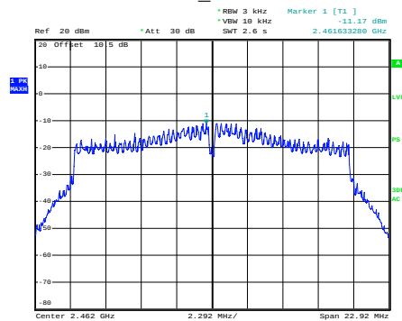
n20_2462MHz
