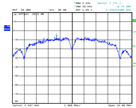
b_2437MHz
