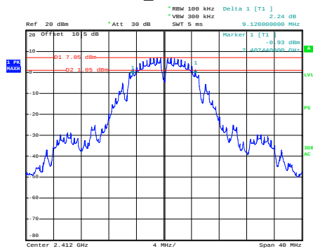
b_2412MHz
