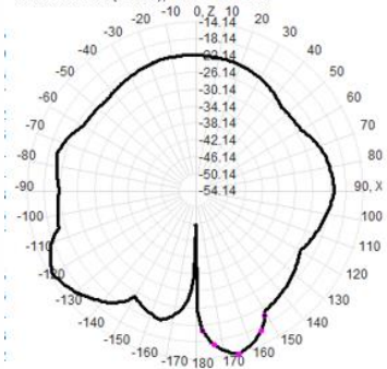
433.0MHz Total(E1-XZ), Max=-14.14dBi
