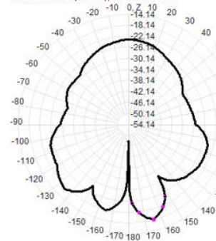
433.0MHz Total(E2-YZ), Max=-18.66dBi
