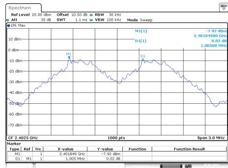
GFSK_Low_DH1
