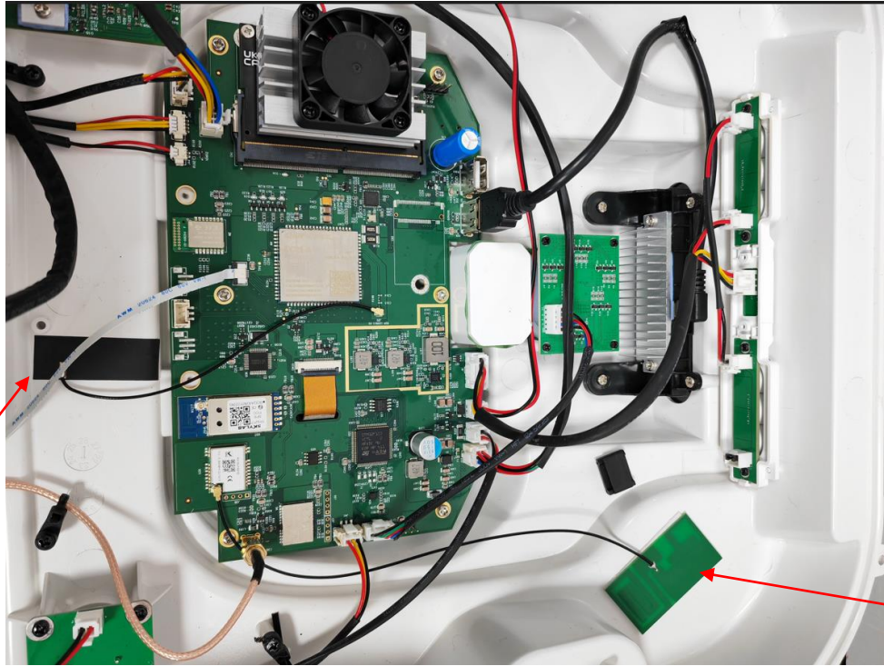
LTE module antenna
