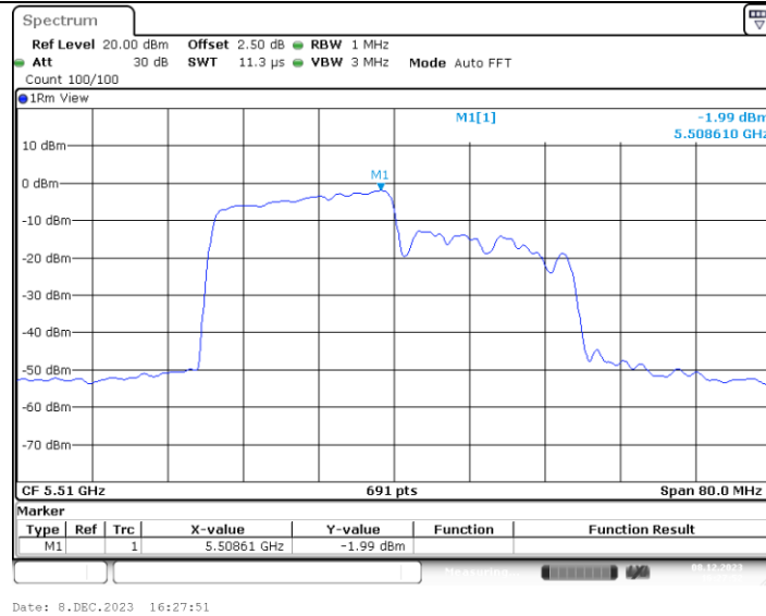
11AX40MIMO Ant1 5510 242Tone RU61
