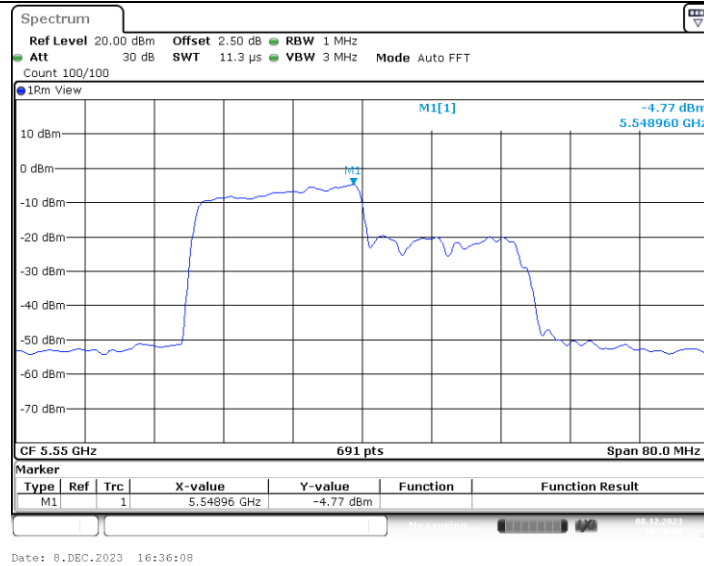
11AX40MIMO Ant4 5550 242Tone RU61
