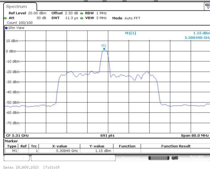
11AX40MIMO Ant3 5310 26Tone RU8
