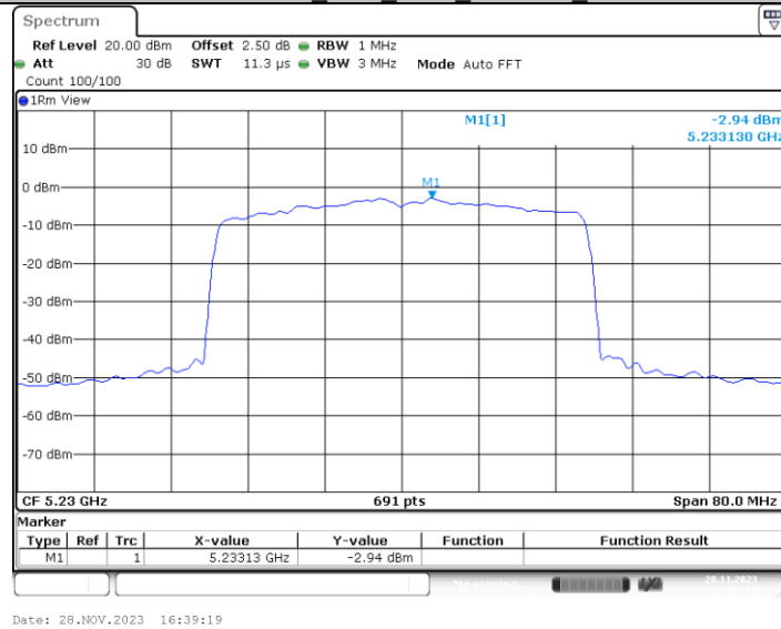
11AX40MIMO Ant1 5230 484Tone RU65
