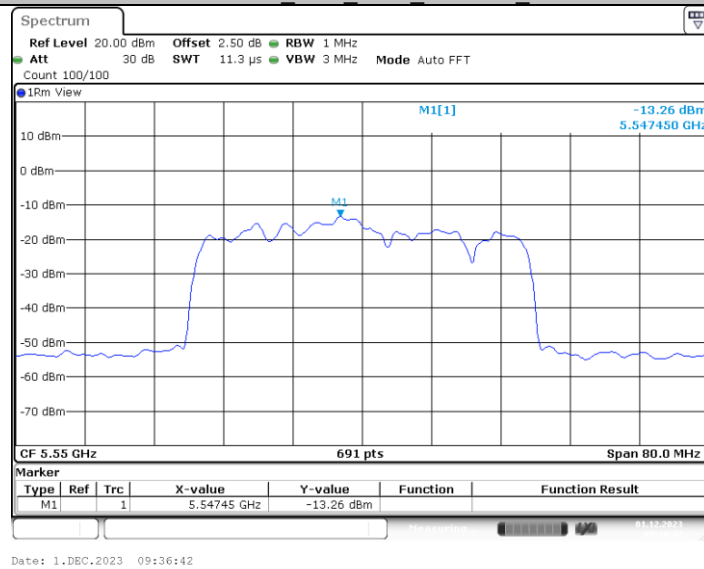
11AX40MIMO Ant4 5550 484Tone RU65
