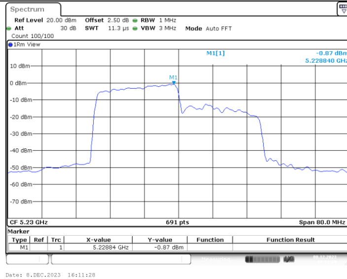
11AX40MIMO Ant1 5230 242Tone RU61
