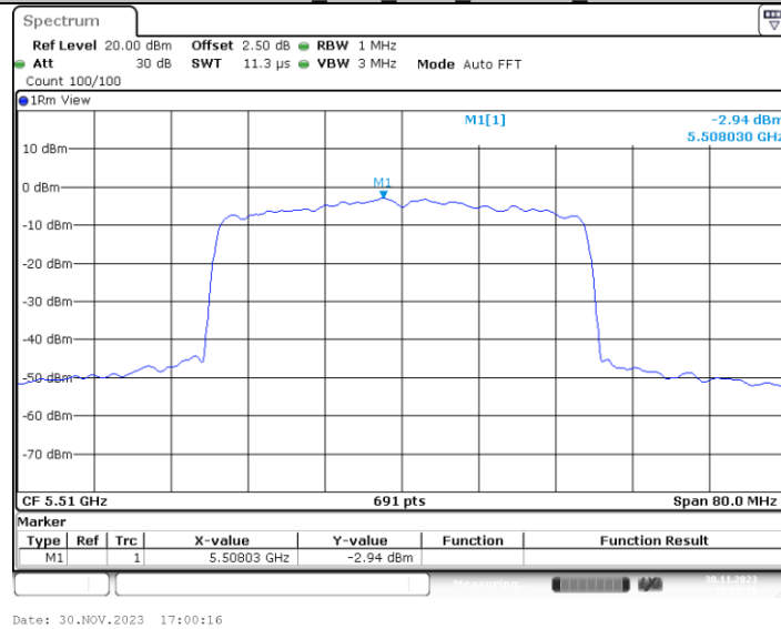
11AX40MIMO Ant1 5510 484Tone RU65
