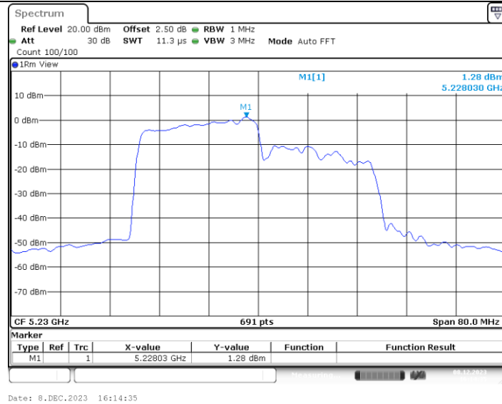
11AX40MIMO Ant4 5230 242Tone RU61
