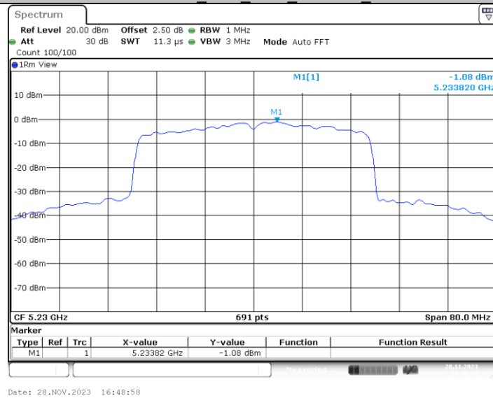
11AX40MIMO Ant4 5230 484Tone RU65
