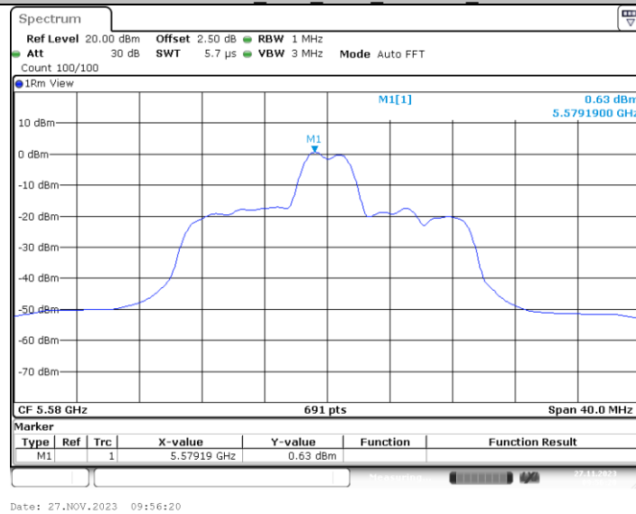
11AX20MIMO_Ant1_5580_26Tone_RU4
