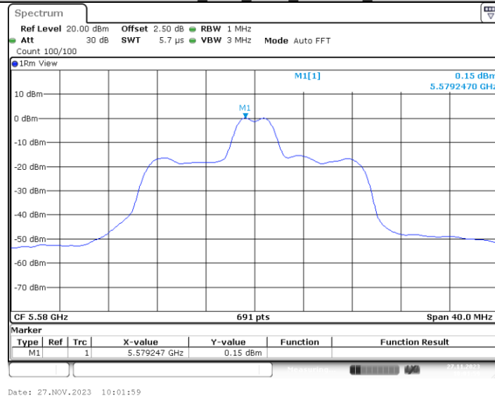
11AX20MIMO_Ant3_5580_26Tone_RU4
