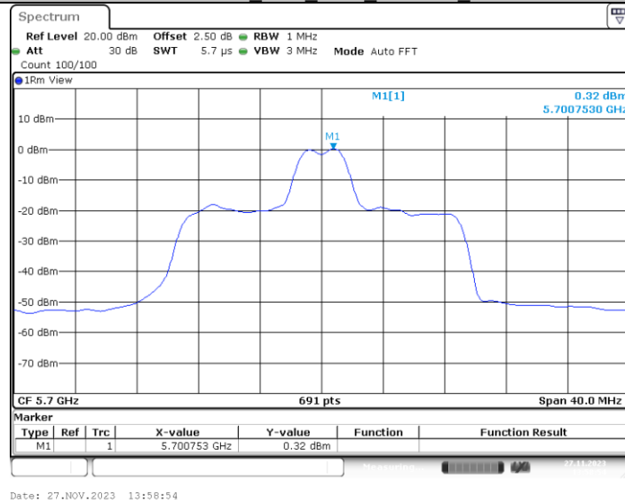
11AX20MIMO_Ant2_5700_26Tone_RU4
