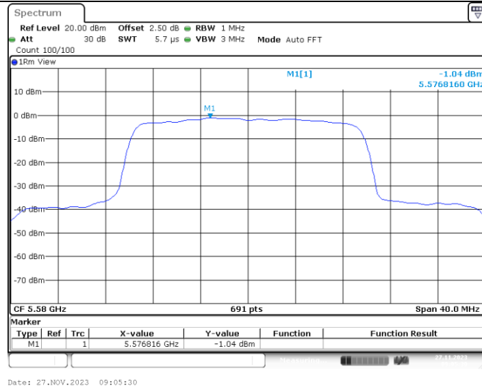
11AX20MIMO_Ant2_5580_242Tone_RU61
