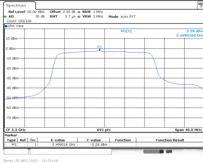
11AX20MIMO_Ant4_5500_242Tone_RU61
