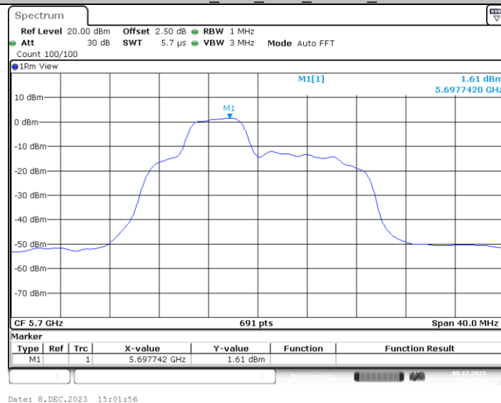
11AX20MIMO_Ant2_5700_52Tone_RU38
