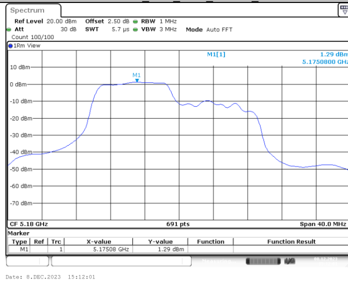
11AX20MIMO_Ant3_5180_106Tone_RU53
