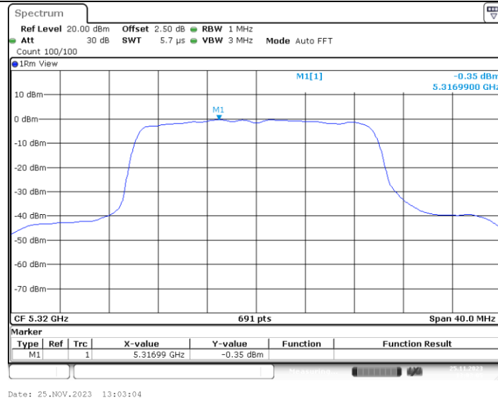
11AX20MIMO_Ant2_5320_242Tone_RU61
