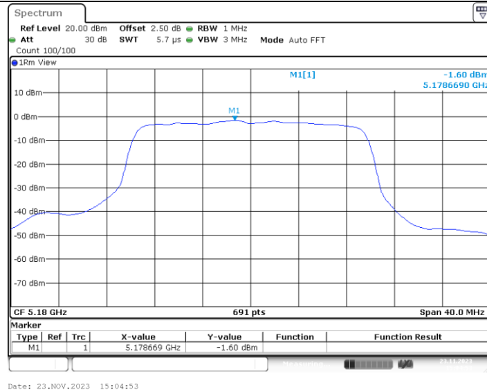
11AX20MIMO_Ant1_5180_242Tone_RU61
