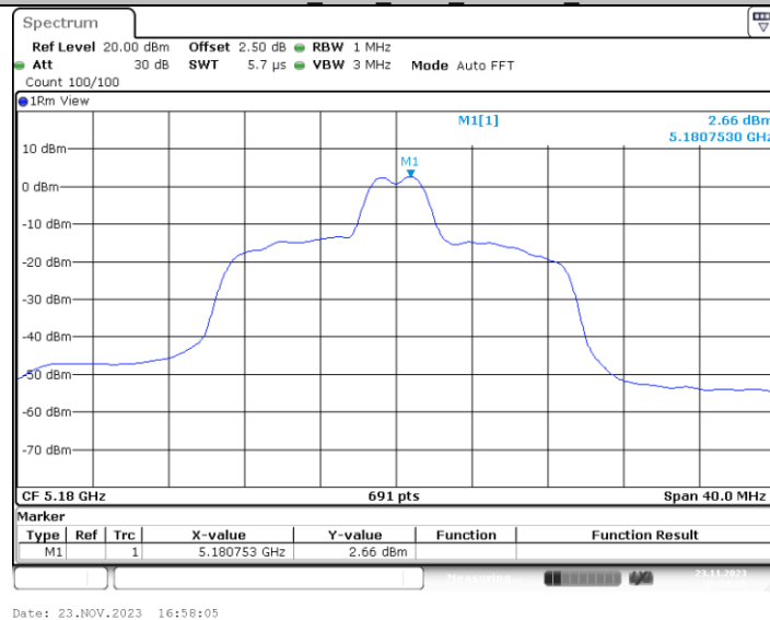
11AX20MIMO_Ant2_5180_26Tone_RU4
