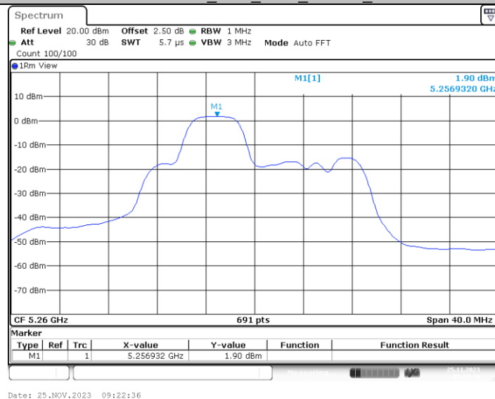
11AX20MIMO_Ant2_5260_52Tone_RU38
