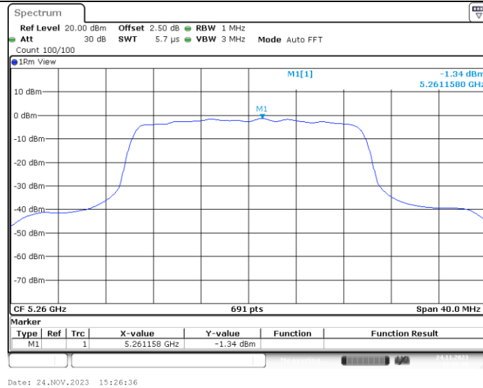
11AX20MIMO_Ant1_5260_242Tone_RU61
