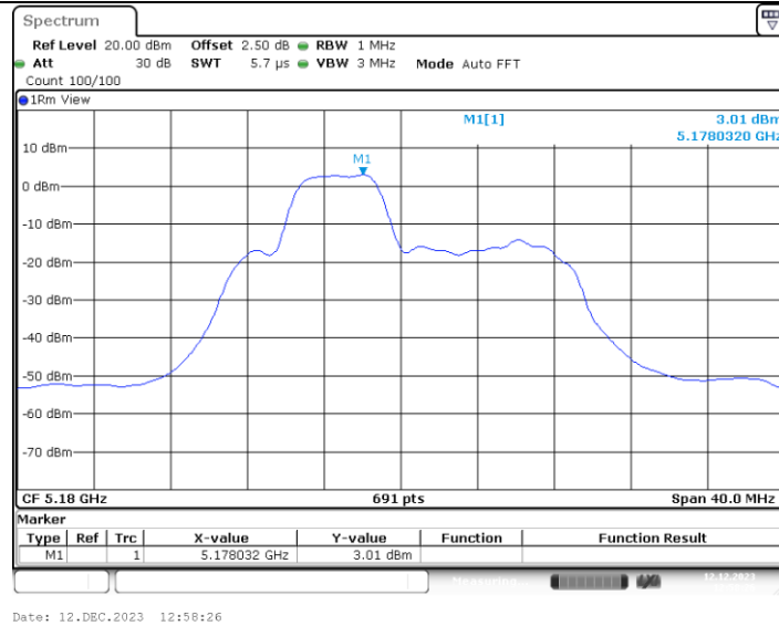
11AX20MIMO_Ant3_5180_52Tone_RU38
