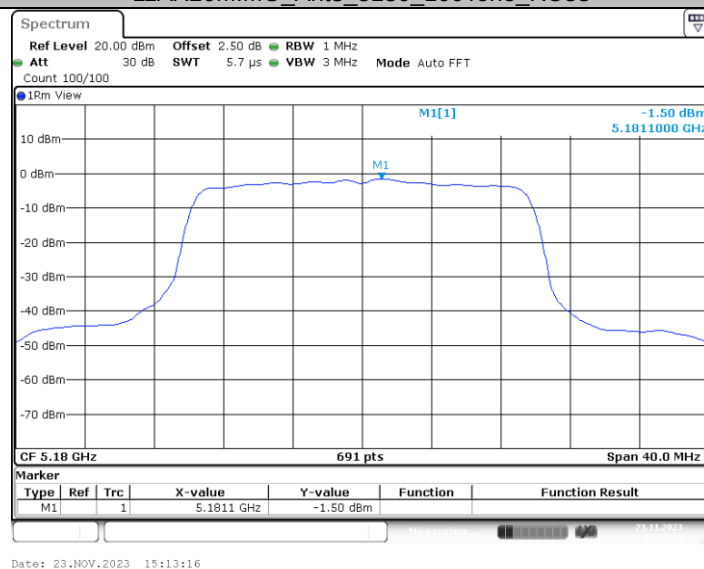
11AX20MIMO_Ant3_5180_242Tone_RU61
