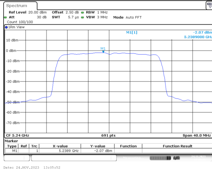
11AX20MIMO_Ant2_5240_242Tone_RU61
