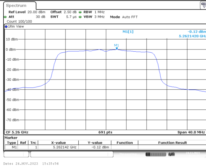
11AX20MIMO_Ant4_5260_242Tone_RU61
