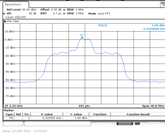
11AX20MIMO_Ant3_5320_26Tone_RU4
