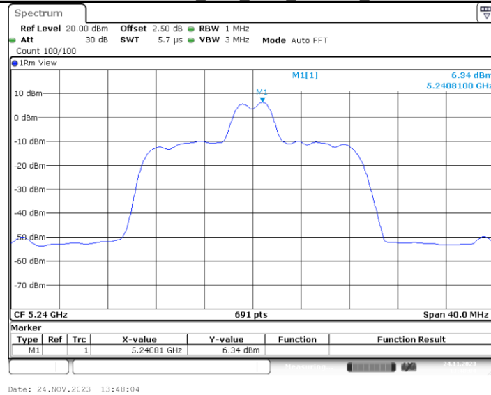
11AX20MIMO_Ant3_5240_26Tone_RU4
