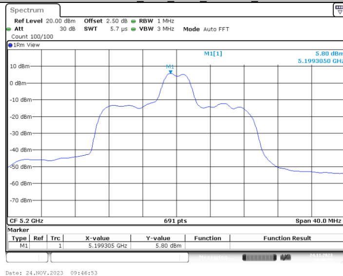
11AX20MIMO_Ant4_5200_26Tone_RU4
