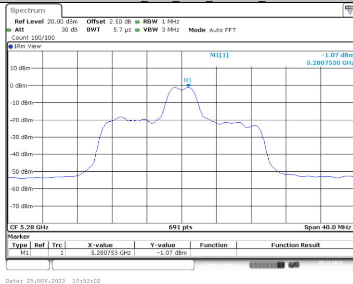
11AX20MIMO_Ant1_5280_26Tone_RU4
