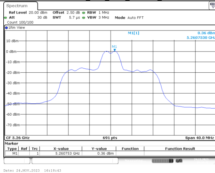
11AX20MIMO_Ant2_5260_26Tone_RU4
