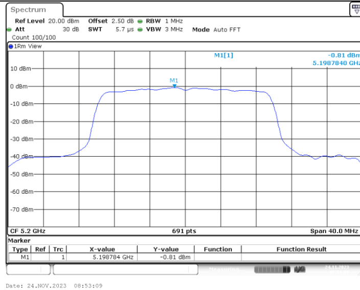
11AX20MIMO_Ant3_5200_242Tone_RU61
