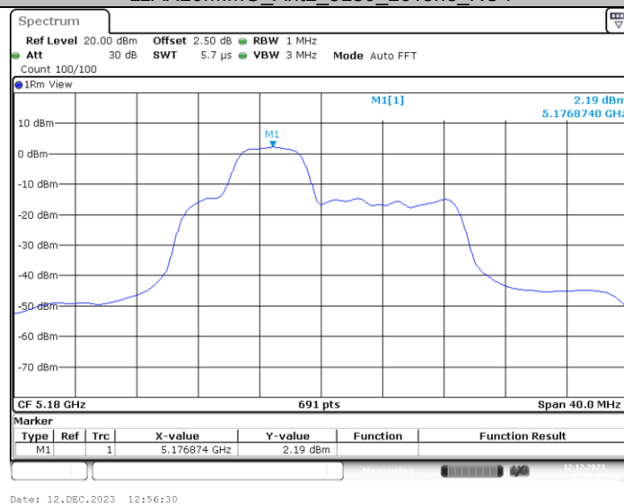
11AX20MIMO_Ant2_5180_52Tone_RU38
