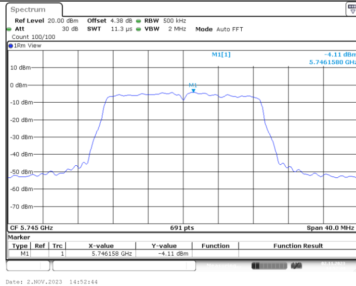
11AC20MIMO_Ant4_5745
