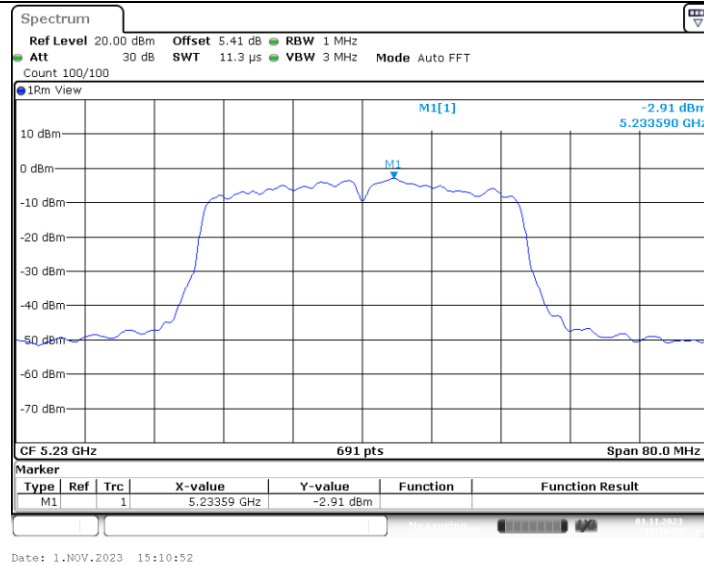
11AC40MIMO_Ant3_5230
