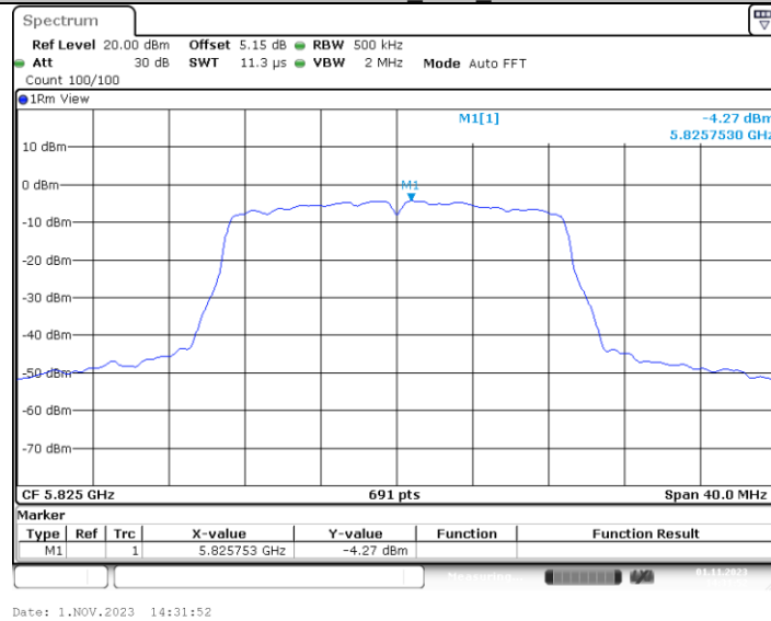
11AC20MIMO_Ant3_5825
