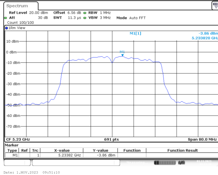
11N40MIMO_Ant3_5230
