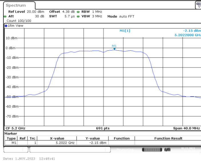
11AC20MIMO_Ant3_5200
