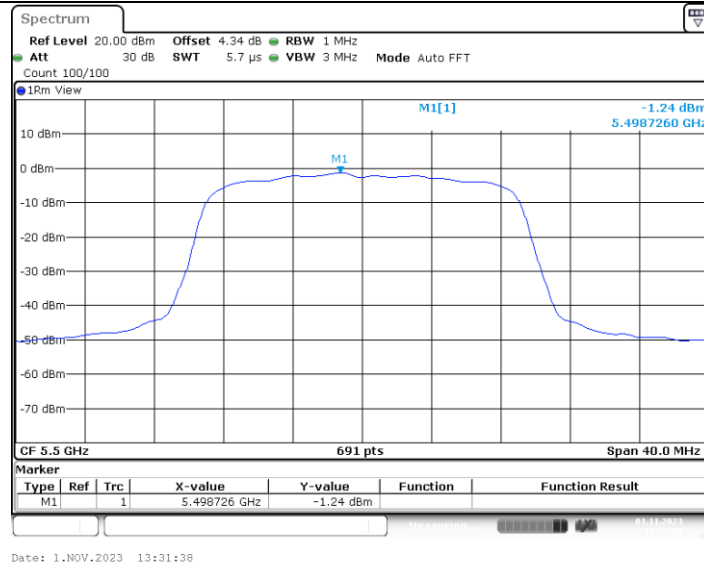
11AC20MIMO_Ant4_5500
