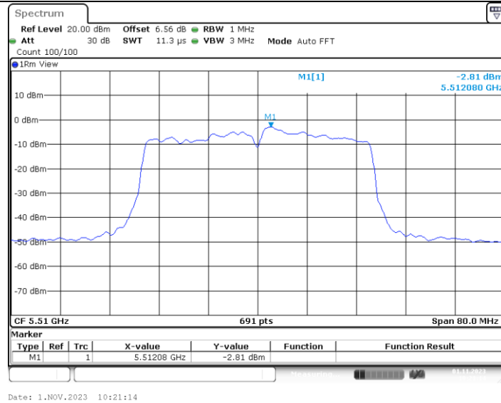
11N40MIMO_Ant3_5510
