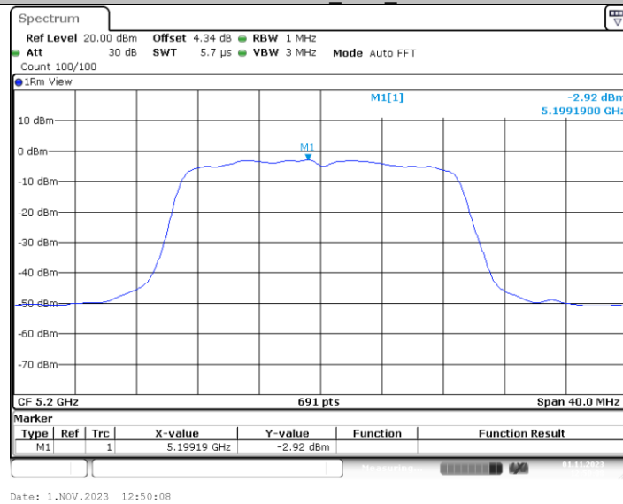
11AC20MIMO_Ant4_5200
