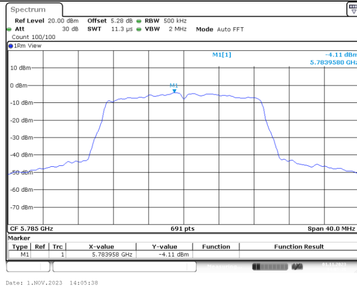
11AC20MIMO_Ant3_5785
