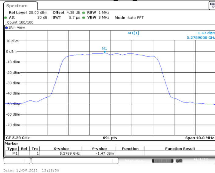
11AC20MIMO_Ant4_5280
