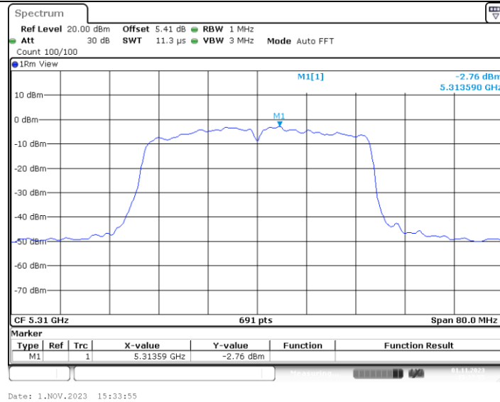
11AC40MIMO_Ant4_5310
