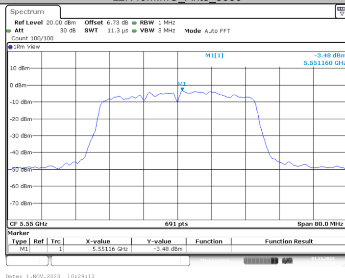
11N40MIMO_Ant4_5550
