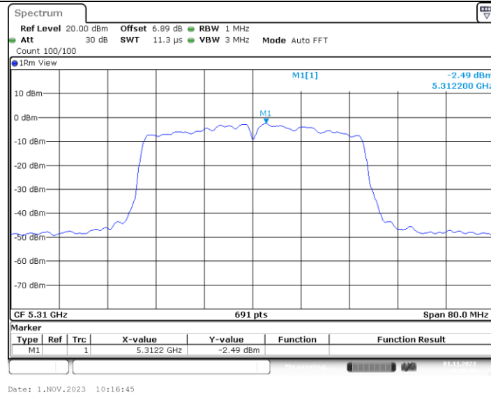
11N40MIMO_Ant4_5310
