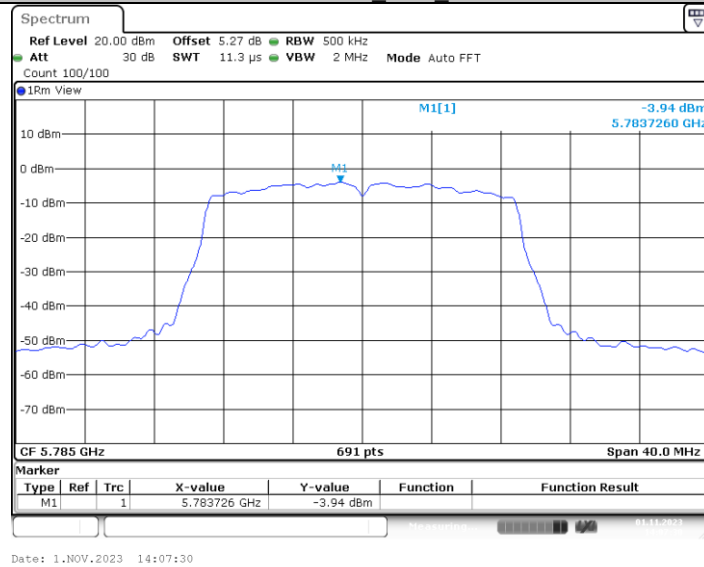
11AC20MIMO_Ant4_5785
