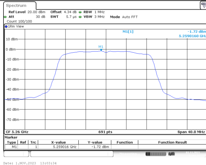
11AC20MIMO_Ant4_5260
