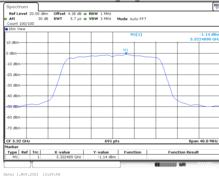
11AC20MIMO_Ant4_5320
