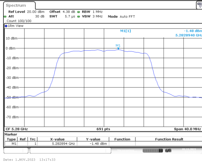
11AC20MIMO_Ant3_5280
