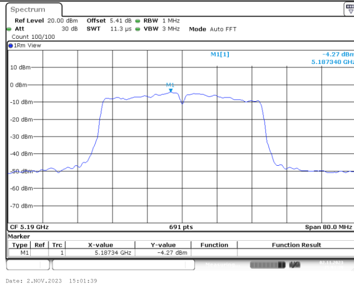
11AC40MIMO_Ant4_5190
