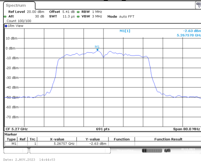
11N40MIMO_Ant3_5270
