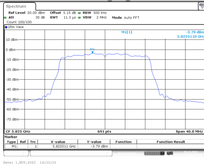
11AC20MIMO_Ant4_5825
