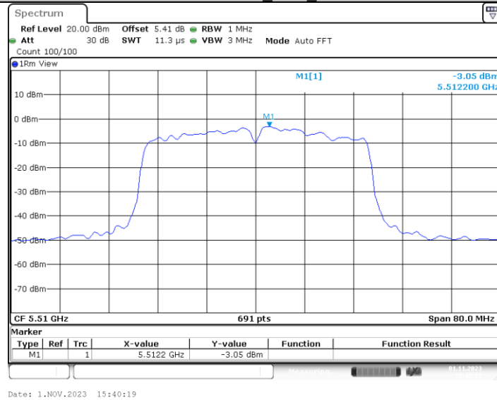
11AC40MIMO_Ant4_5510
