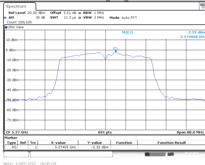
11N40MIMO_Ant4_5270
