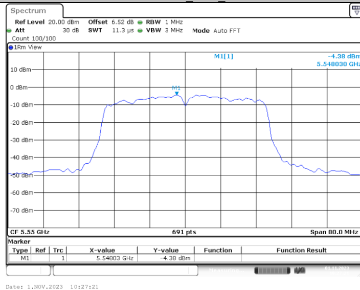
11N40MIMO_Ant3_5550
