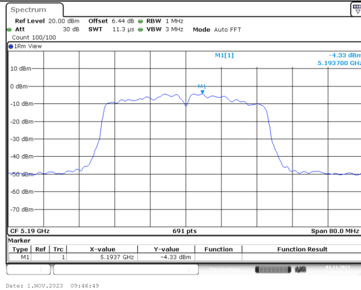
11N40MIMO_Ant4_5190
