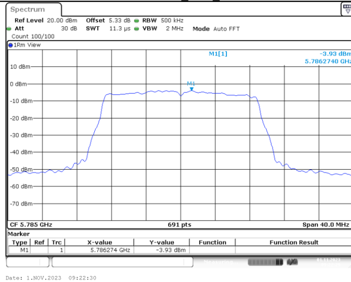
11N20MIMO_Ant4_5785
