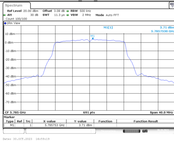
11A_Ant2_5785
