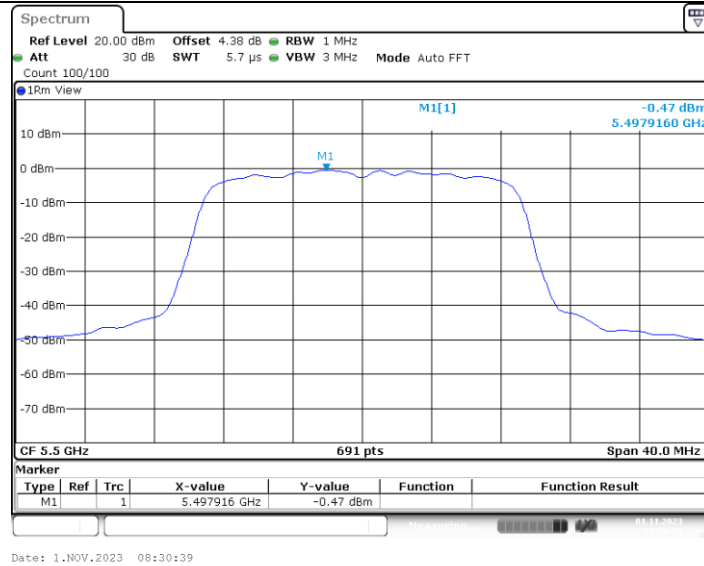
11N20MIMO_Ant4_5500
