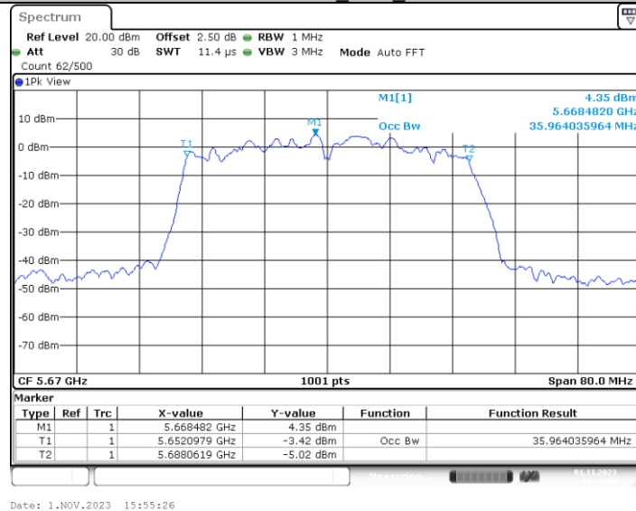
11AC40MIMO_Ant4_5670
