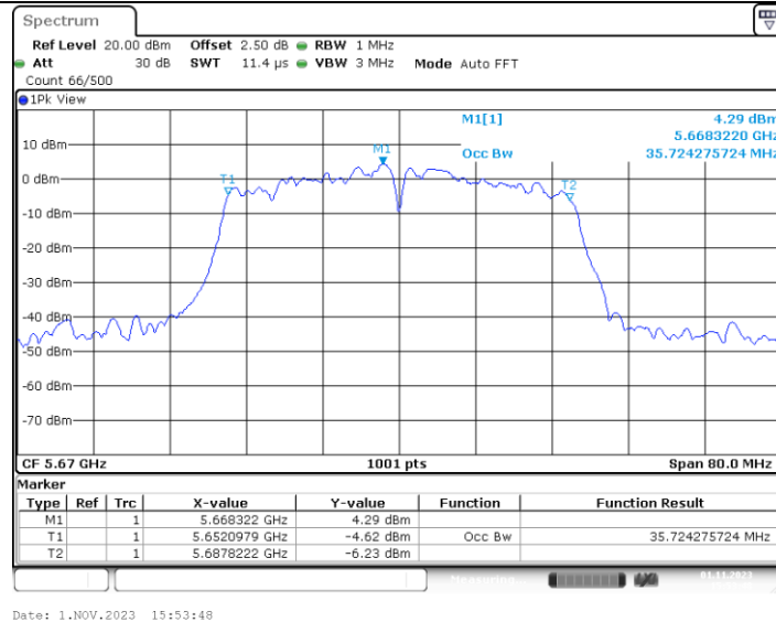
11AC40MIMO_Ant3_5670
