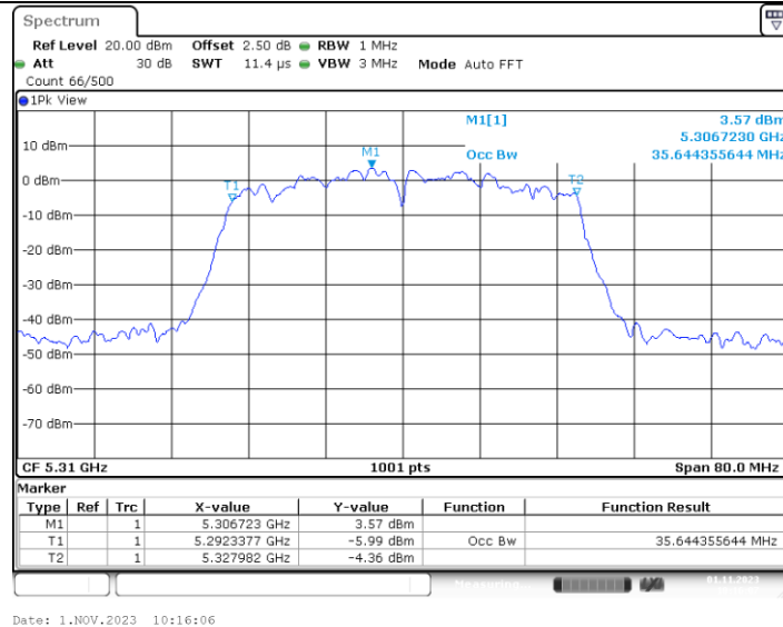
11N40MIMO_Ant3_5310
