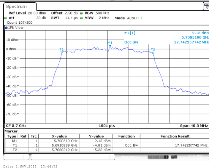
11AC20MIMO_Ant3_5700
