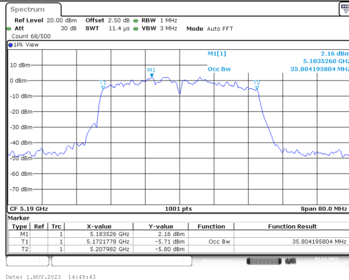
11AC40MIMO_Ant3_5190
