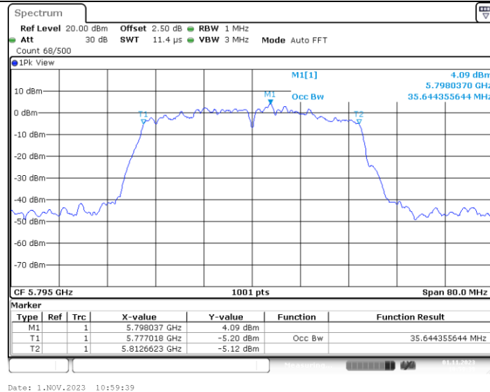
11N40MIMO_Ant4_5795
