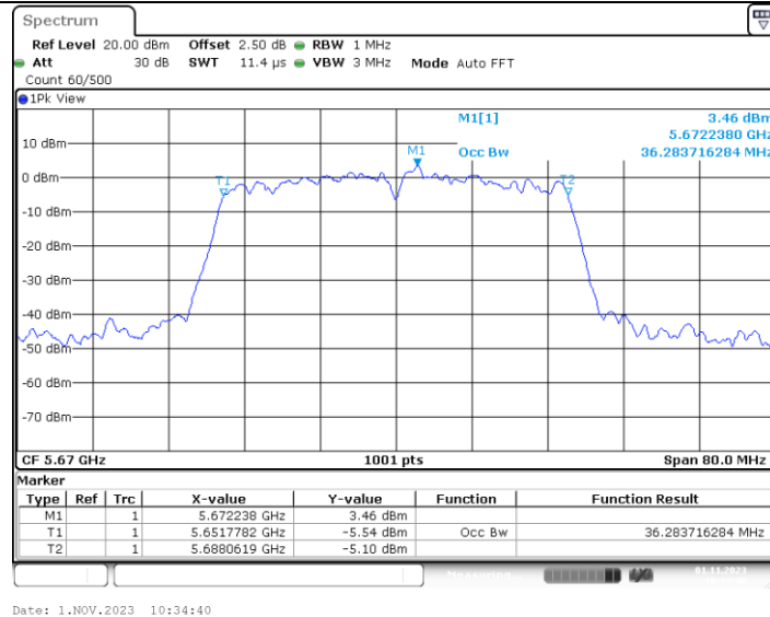
11N40MIMO_Ant3_5670
