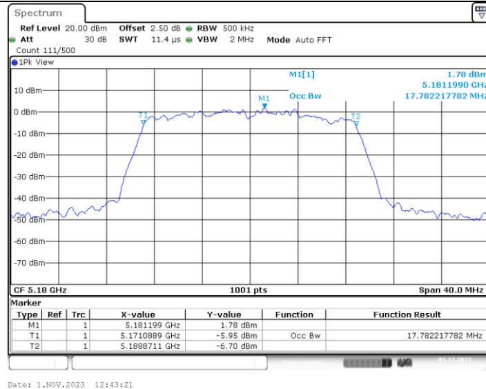
11AC20MIMO_Ant3_5180
