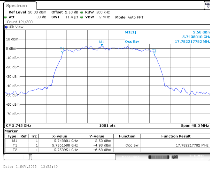
11AC20MIMO_Ant3_5745
