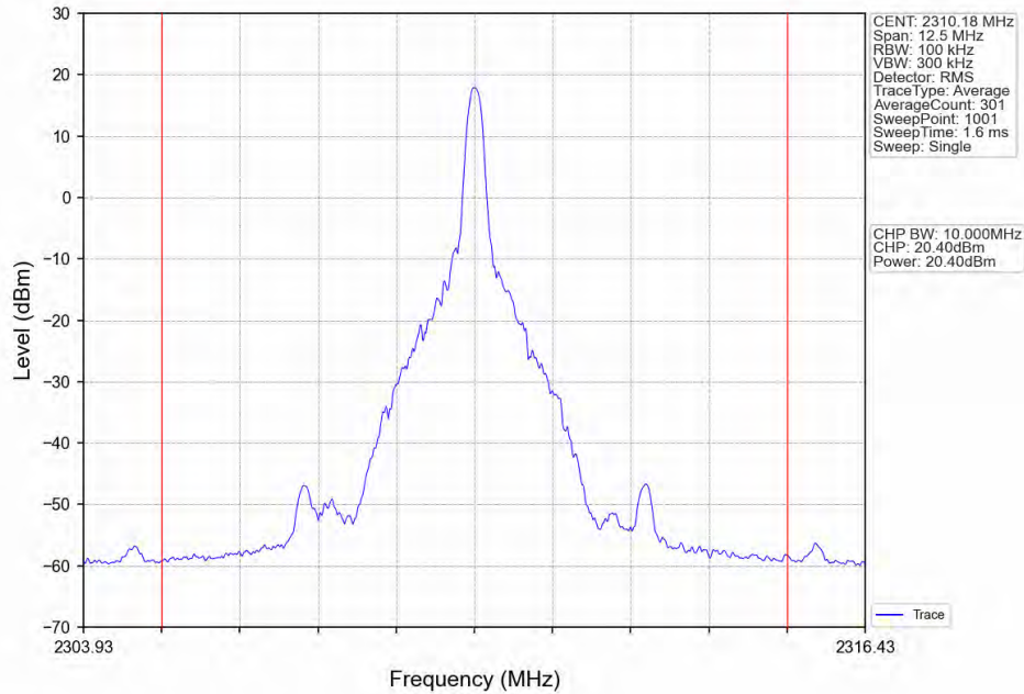
Band30_5MHz_QPSK_MCH_2310MHz_RB_1_24_NTNV
