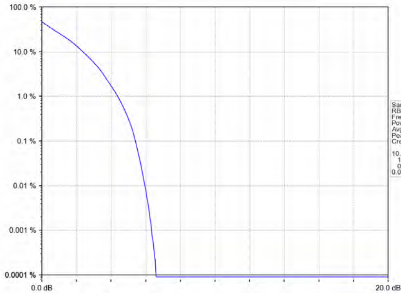
Band4_20MHz_QPSK_MCH_1732.5MHz_RB_100_0_NTNV
