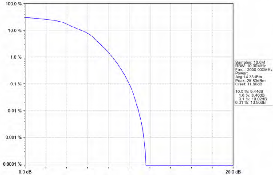
Band43 10MHz 16QAM MCH 3650MHz RB 50_0 NTN
