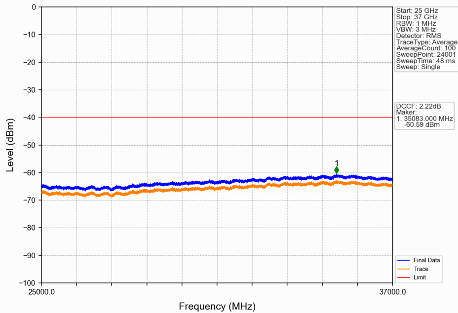
Band48_15MHz_QPSK_HCH_3692.5MHz_RB_1_74_NTNV
