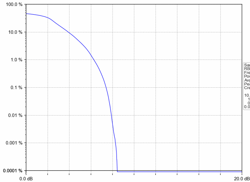
Band48_10MHz_QPSK_HCH_3695MHz_RB_50_0_NTNV
