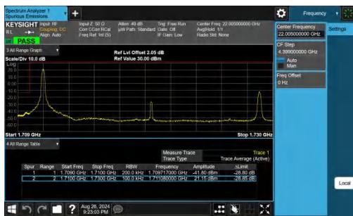
Band66-20MHz-QPSK-132072-1RB#0-PASS
