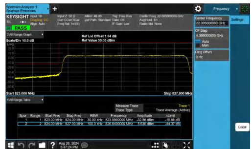
Band26(824-849)-3MHz-QPSK-26805-15RB#0-PASS
