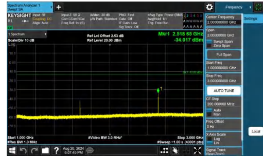
Band26(824-849)-10MHz-QPSK-26990-1RB#0-1000~3000-PASS
