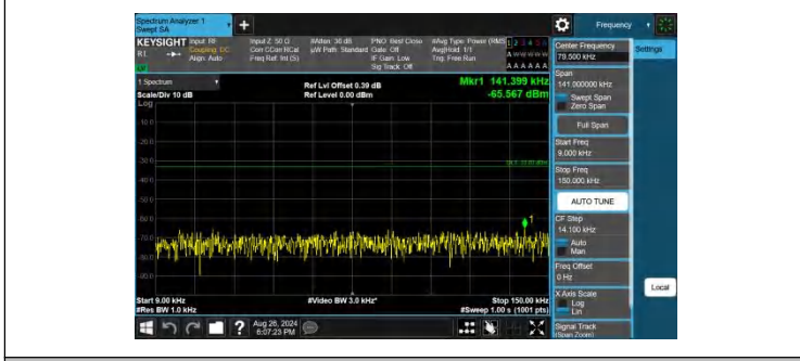
Band26(824-849)-10MHz-QPSK-26990-1RB#0-0.009~0.15-PASS
