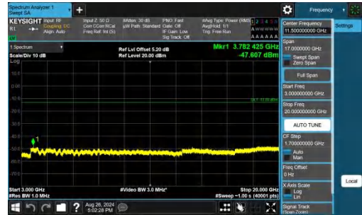
Band25-20MHz-QPSK-26365-1RB#99-3000~20000-PASS
