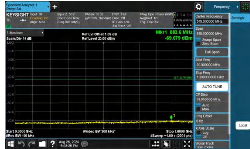
Band25-20MHz-QPSK-26590-1RB#99-30~1000-PASS
