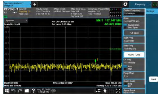
Band25-10MHz-QPSK-26365-1RB#49-0.009~0.15-PASS
