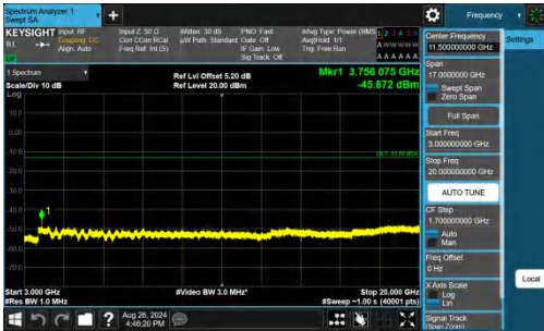
Band25-10MHz-QPSK-26365-1RB#0-3000~20000-PASS
