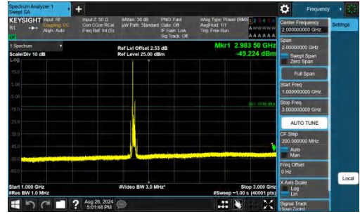
Band25-20MHz-QPSK-26365-1RB#0-1000~3000-PASS
