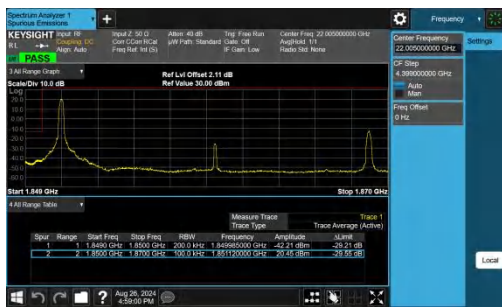
Band25-20MHz-QPSK-26140-1RB#0-PASS
