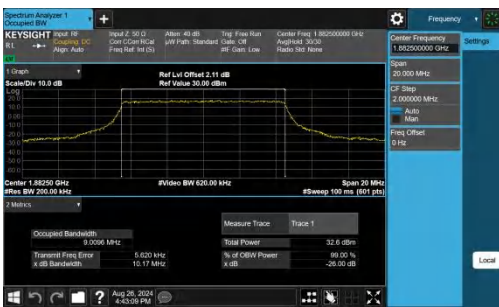
Band25-10MHz-QPSK-26365-50RB#0-PASS
