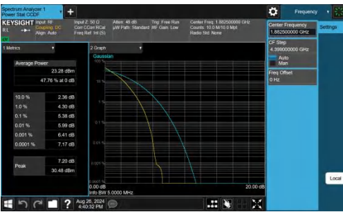
Band25-5MHz-QPSK-26365-25RB#0-PASS
