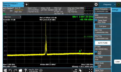
Band25-20MHz-QPSK-26590-1RB#0-1000~3000-PASS
