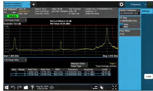
Band25-20MHz-QPSK-26590-1RB#99-PASS
