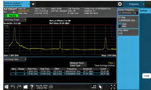
Band25-20MHz-QPSK-26590-1RB#0-PASS
