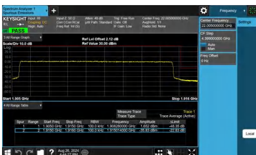
Band25-10MHz-QPSK-26640-50RB#0-PASS
