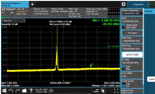
Band25-20MHz-QPSK-26365-1RB#99-1000~3000-PASS
