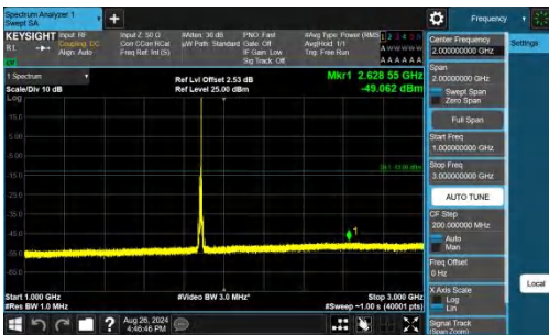
Band25-10MHz-QPSK-26365-1RB#49-1000~3000-PASS
