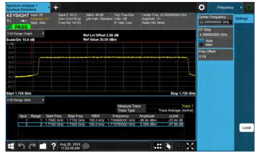
Band4-10MHz-QPSK-20000-50RB#0-PASS
