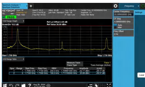
Band4-20MHz-QPSK-20050-1RB#0-PASS
