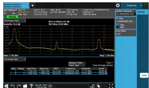
Band4-10MHz-QPSK-20350-1RB#0-PASS
