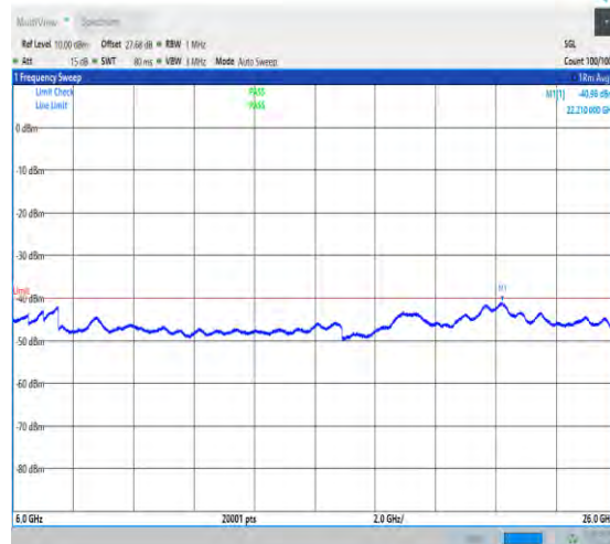
NTVN_N48_PC3_30_40_L_TID1_NS_01_6000_26000_#1
