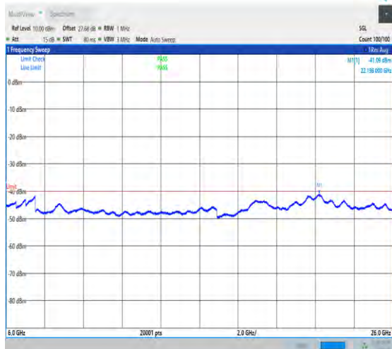
NTVN_N48_PC3_30_40_M_TID1_NS_01_6000_26000_#
