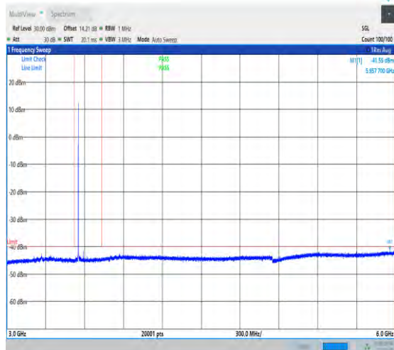
NTVN_N48_PC3_30_40_L_TID1_NS_01_3000_6000_#1
