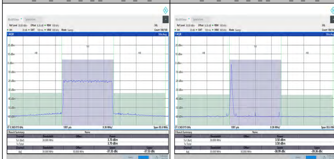
NTNV_N48_PC3_30_30_L_TID19_#1_-30_30
