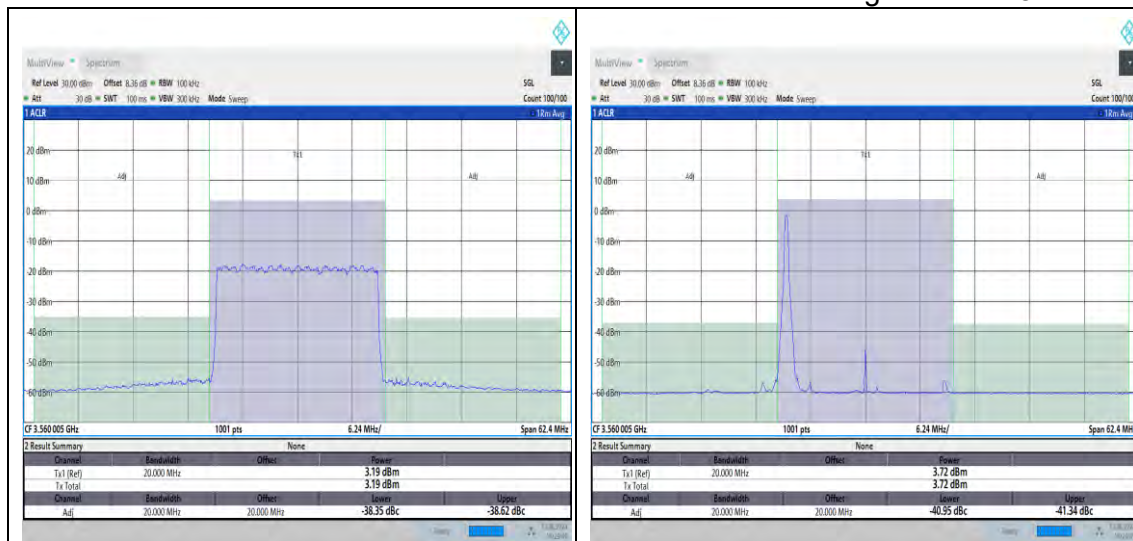
NTNV_N48_PC3_30_20_L_TID22_#1_-20_20
