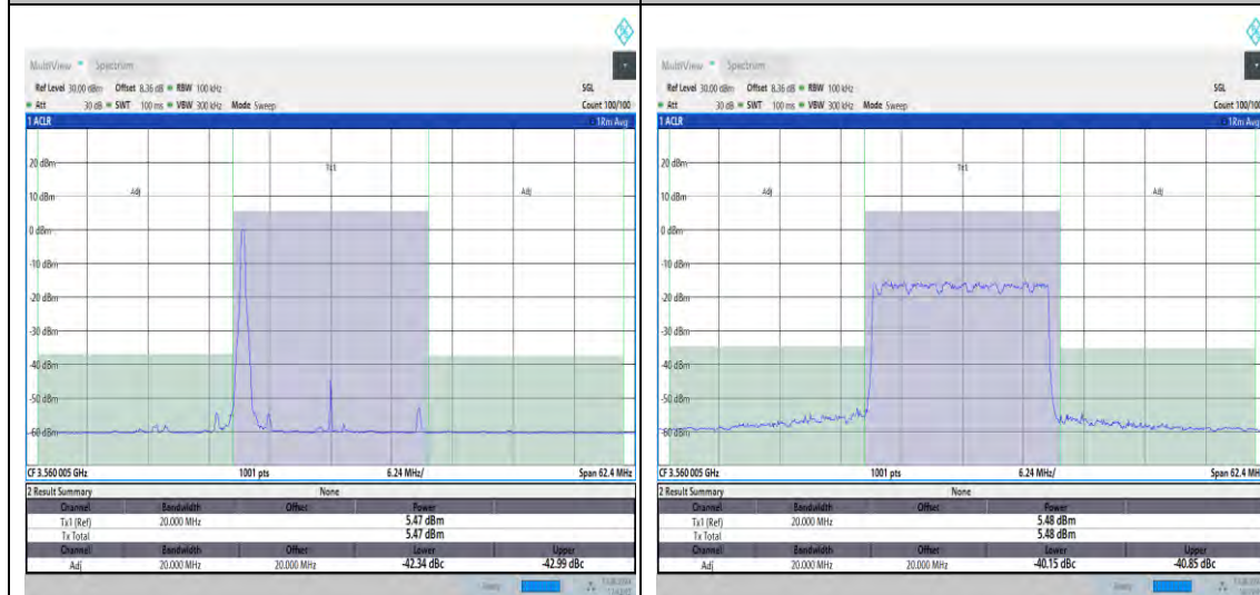
NTNV_N48_PC3_30_20_L_TID2_#1_+20_20
