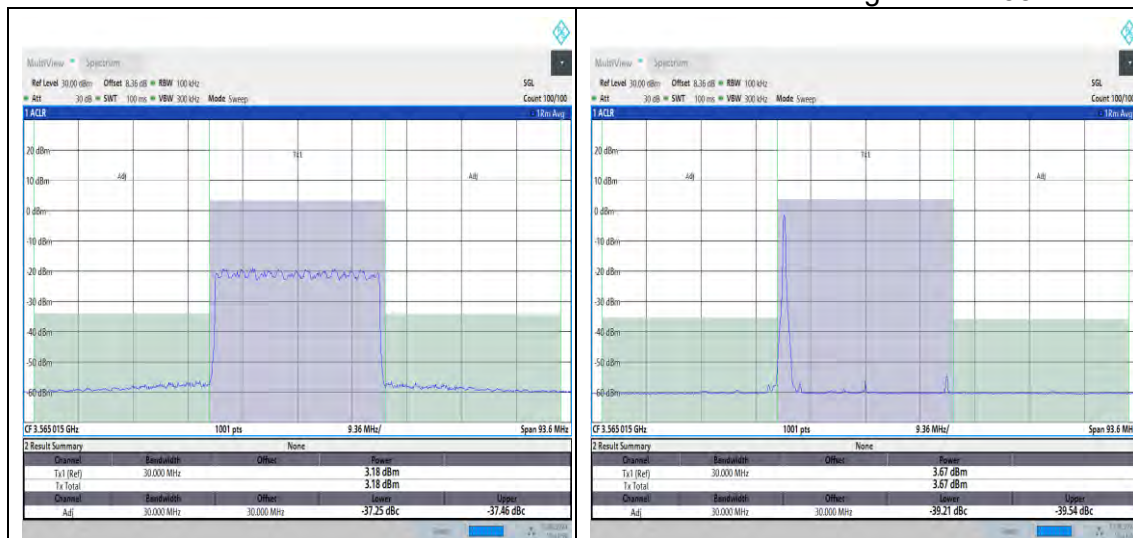
NTNV_N48_PC3_30_30_L_TID22_#1_-30_30
