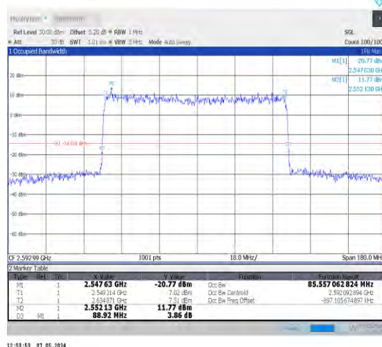
1-N41-30-90-M-5-DFT-256QAM-Outer_Full-240@0-A Ant0-85.557-88.920-≤90-PASS
