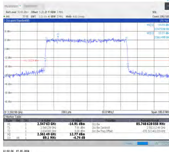
1-N41-30-90-M-3-DFT-16QAM-Outer_Full-240@0-A nt0-85.749-89.100-≤90-PASS
