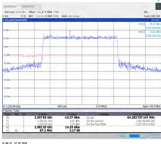
1-N41-30-70-M-4-DFT-64QAM-Outer_Full-180@0-A nt0-64.284-67.200-≤70-PASS
