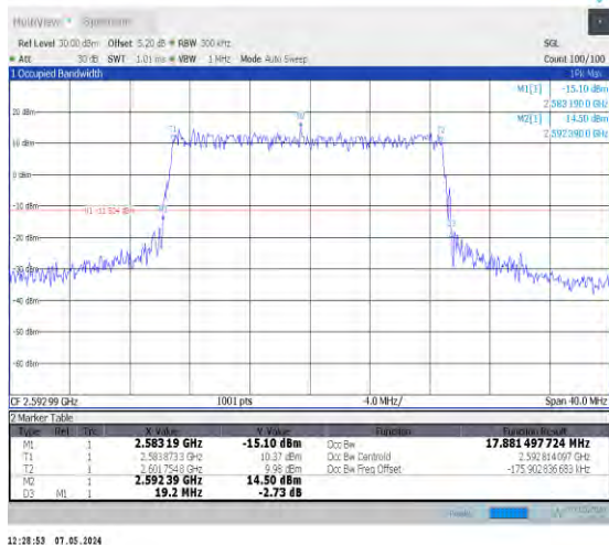
1-N41-30-20-M-3-DFT-16QAM-Outer_Full-50@0-Ant0 0-17.881-19.200-≤20-PASS
