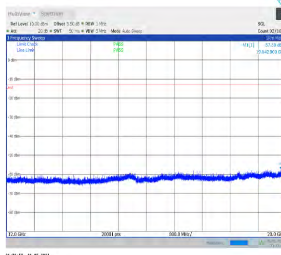
1-N14-PC3-15-10-M-1-DFT-PI2BPSK-Inner_1RB_L ef t-1@1-12000-20000-Ant0-19842.80--57.58--13-PASS
