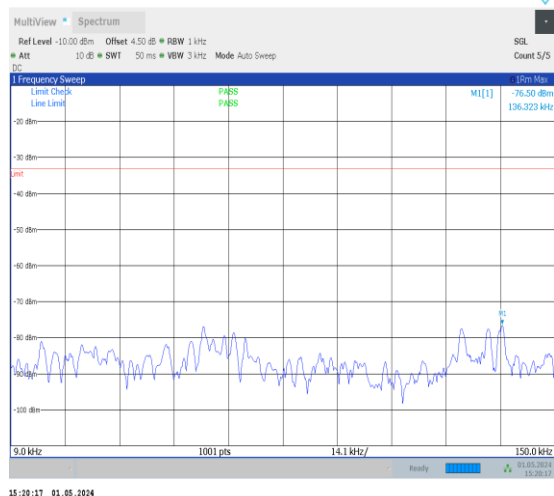
1-N13-PC3-15-10-M-1-DFT-PI2BPSK-Inner_1RB_L eft-1@1-0.009-0.15-Ant0-0.14--76.50--33-PASS
