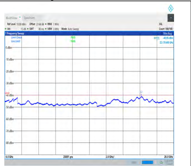
NTVN_N48_PC3_30_40_L_TID1_NS_01_6000_26000_#1
