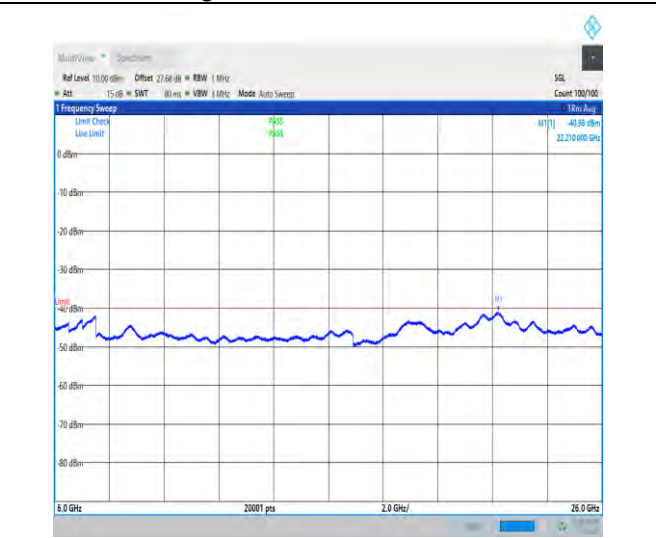
NTVN_N48_PC3_30_40_L_TID1_NS_01_6000_26000_#1
