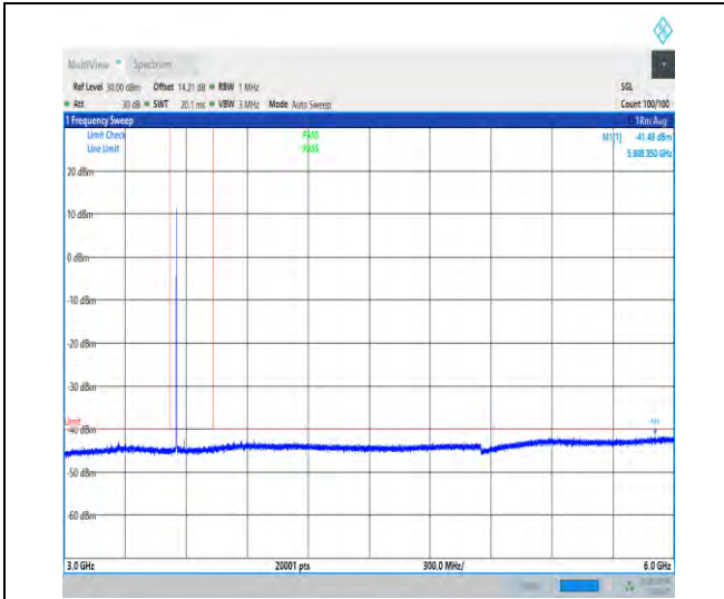
NTVN_N48_PC3_30_40_L_TID1_NS_01_3000_6000_#1
