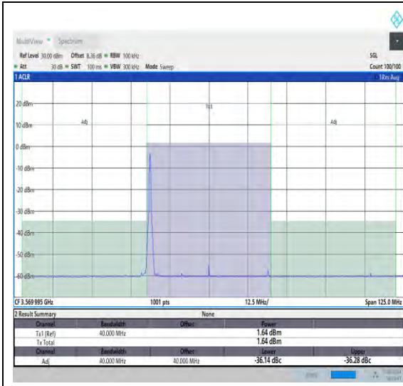
NTNV_N48_PC3_30_40_L_TID26_#1_40_40
