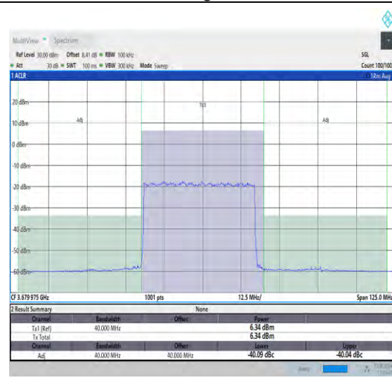
NTNV_N48_PC3_30_40_H_TID1_#1_40_40
