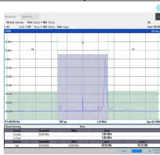
NTNV_N48_PC3_30_20_H_TID6 #1_+20_20
