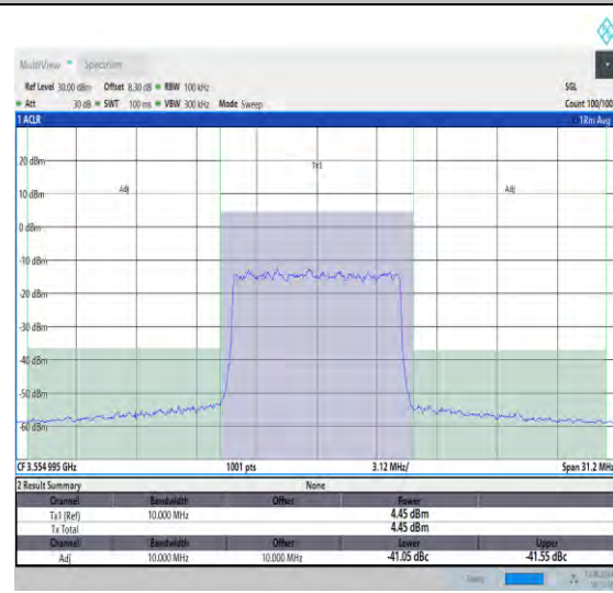
NTVN_N48_PC3_30_10_L_TID7_#1_-10_10
