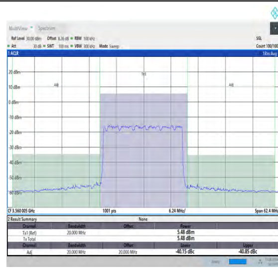
NTNV_N48_PC3_30_20_L_TID4_#1_-20_20
