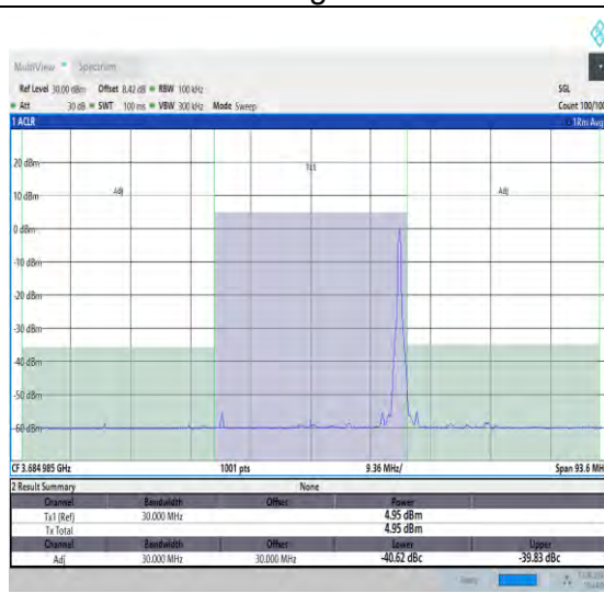
NTNV_N48_PC3_30_30_H_TID3_#1_-30_30
