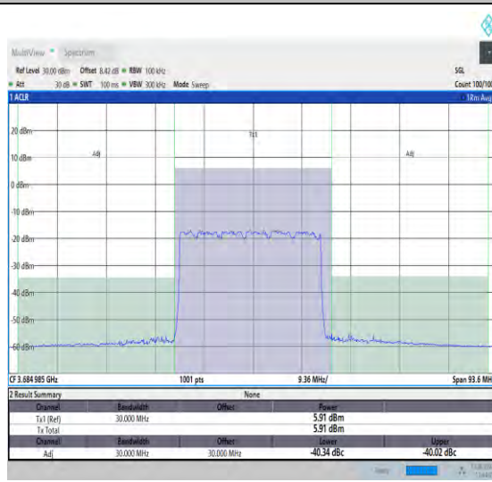
NTNV_N48_PC3_30_30_H_TID4_#1_+30_30
