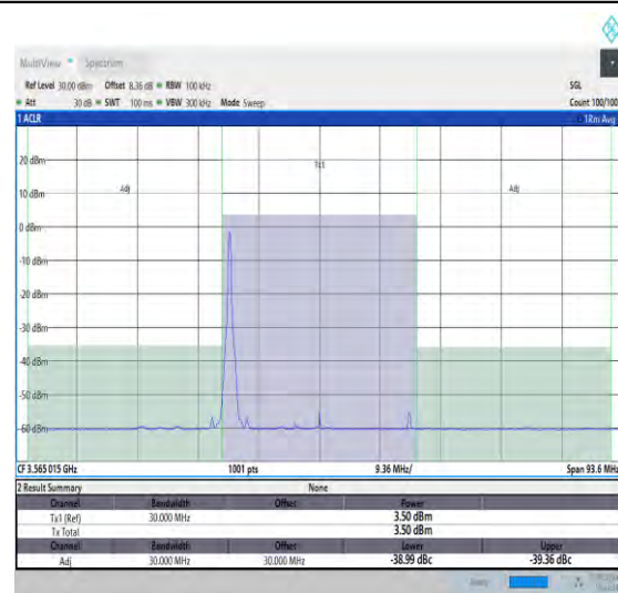
NTNV_N48_PC3_30_30_L_TID20_#1_-30_30
