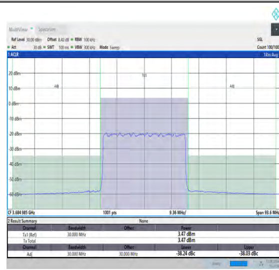
NTNV_N48_PC3_30_30_H_TID22_#1_-30_30
