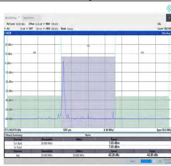
NTNV_N48_PC3_30_30_L_TID5_#1_-30_30
