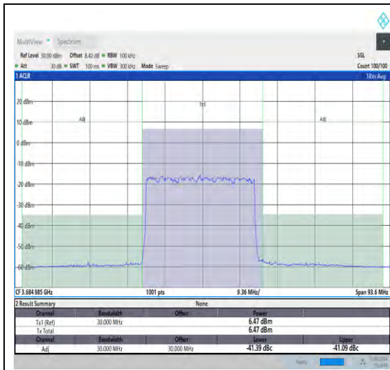
NTNV_N48_PC3_30_30_H_TID1_#1_-30_30
