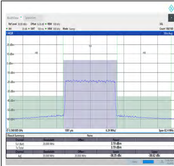
NTNV_N48_PC3_30_20_L_TID22_#1_-20_20
