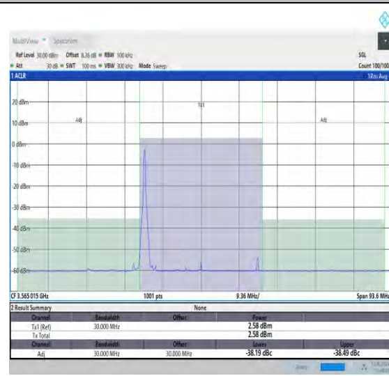
NTNV_N48_PC3_30_30_L_TID14_#1_-30_30
