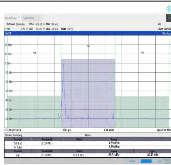
NTNV_N48_PC3_30_30_L_TID8_#1_-30_30
