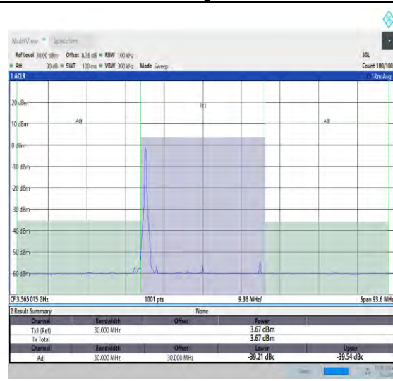
NTNV_N48_PC3_30_30_L_TID23_#1_-30_30
