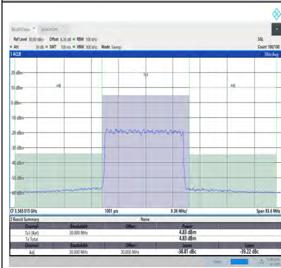
NTNV_N48_PC3_30_30_L_TID7_#1_-30_30
