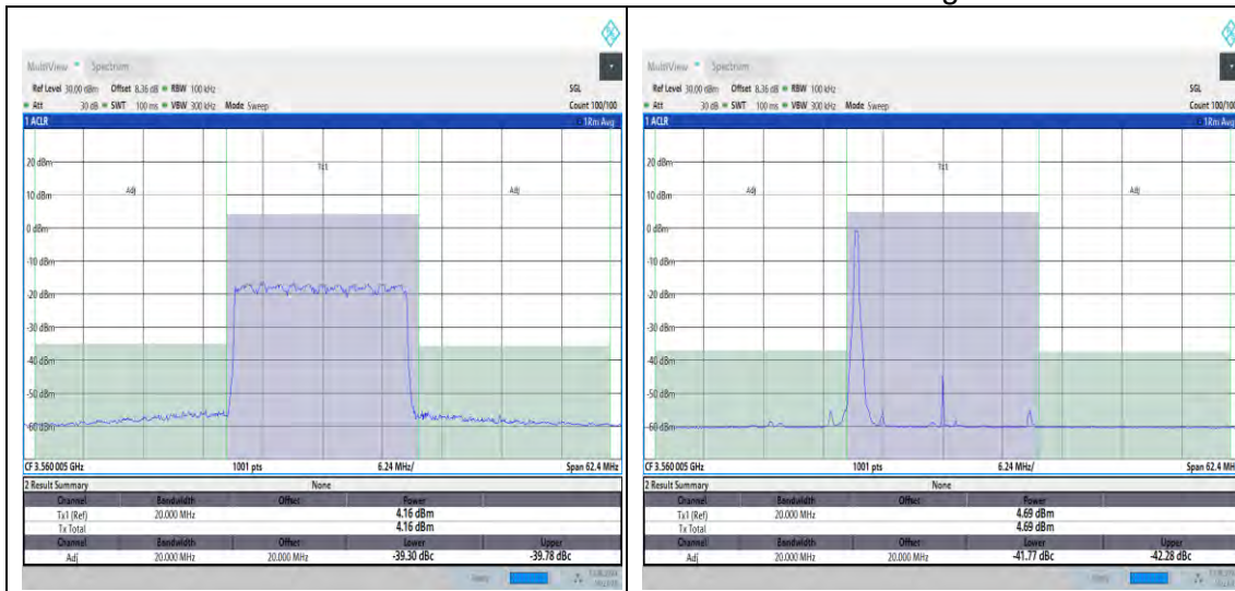
NTNV_N48_PC3_30_20_L_TID10_#1_-20_20
