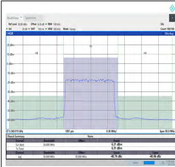
NTVN_N48_PC3_30_30_L_TID1_#1_-30_30
