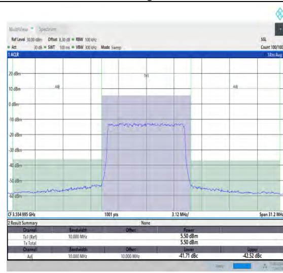
NTVN_N48_PC3_30_10_L_TID4_#1_+10_10
