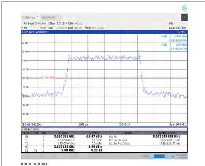
1-N48-30-10-M-9-CP-256QAM-Outer_Full-24@0-Ant 0-8.563-9.080-≤10-PASS
