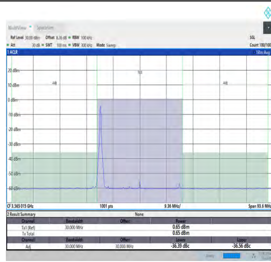
NTNV_N48_PC3_30_30_L_TID26_#1_-30_30
