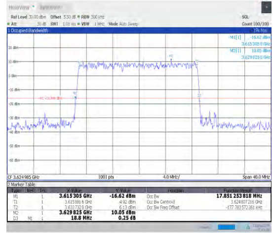
1-N48-30-20-M-5-DFT-256QAM-Outer_Full-50@0-A nt0-17.851-18.800-≤20-PASS
