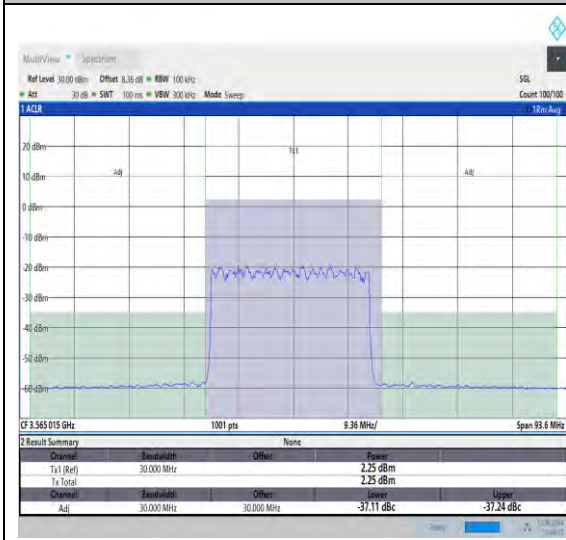
NTNV_N48_PC3_30_30_L_TID13_#1_-30_30
