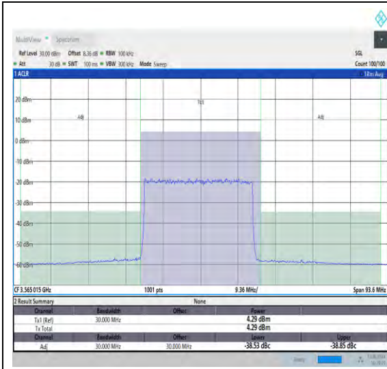
NTNV_N48_PC3_30_30_L_TID10_#1_-30_30
