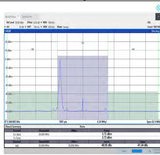
NTNV_N48_PC3_30_20_L_TID23_#1_-20_20
