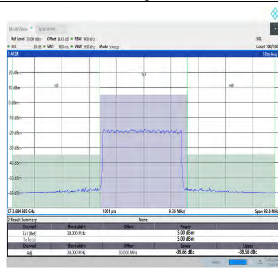
NTNV_N48_PC3_30_30_H_TID7_#1_30_30
