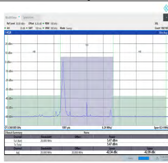
NTNV_N48_PC3_30_20_L_TID2_#1_-20_20
