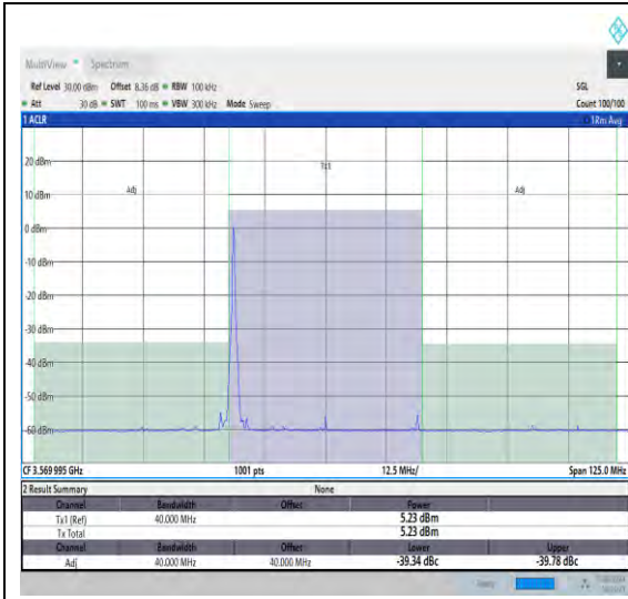
NTNV_N48_PC3_30_40_L_TID8_#1_-40_40
