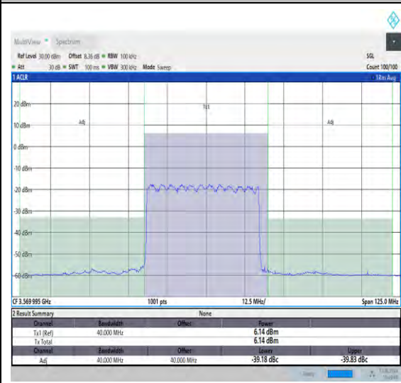
NTNV_N48_PC3_30_40_L_TID1_#1_-40_40
