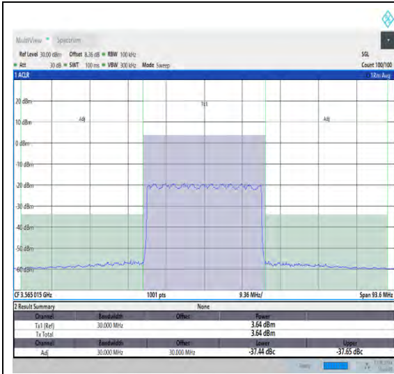
NTNV_N48_PC3_30_30_L_TID16_#1_-30_30
