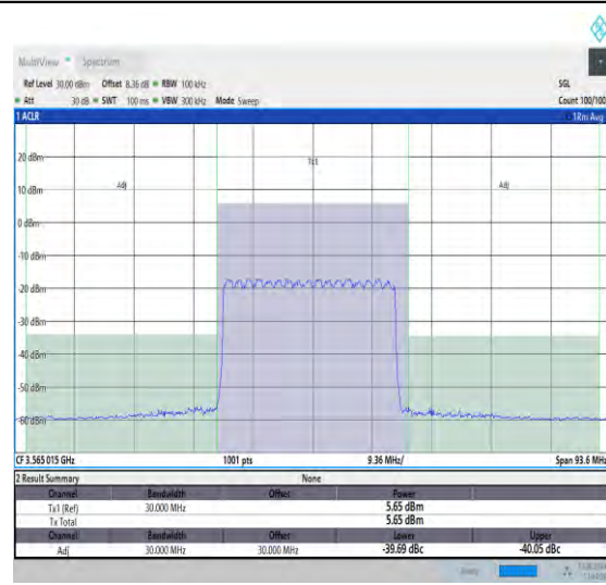
NTVN_N48_PC3_30_30_L_TID4_#1_-30_30
