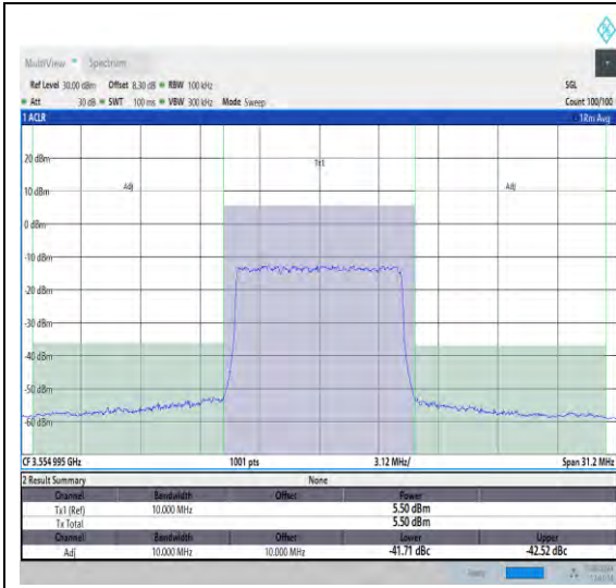
NTVN_N48_PC3_30_10_L_TID4_#1_-10_10
