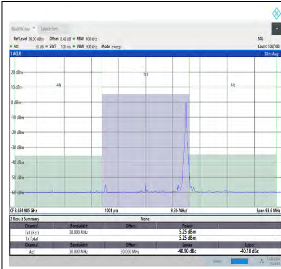
NTNV_N48_PC3_30_30_H_TID6_#1_30_30
