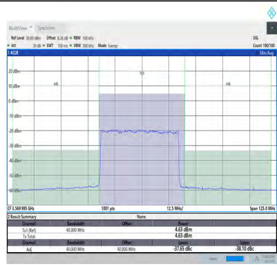
NTVN_N48_PC3_30_40_L_TID7_#1_-40_40
