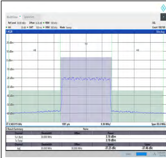
NTNV_N48_PC3_30_30_L_TID22_#1_-30_30
