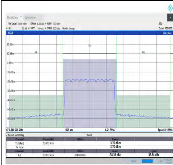
NTNV_N48_PC3_30_20_L_TID19_#1_-20_20
