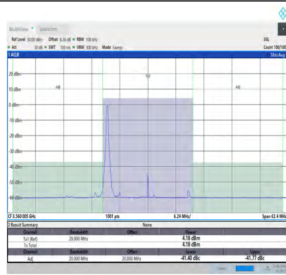
NTNV_N48_PC3_30_20_L_TID20_#1_-20_20
