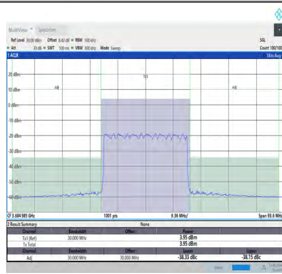
NTNV_N48_PC3_30_30_H_TID16_#1_30_30
