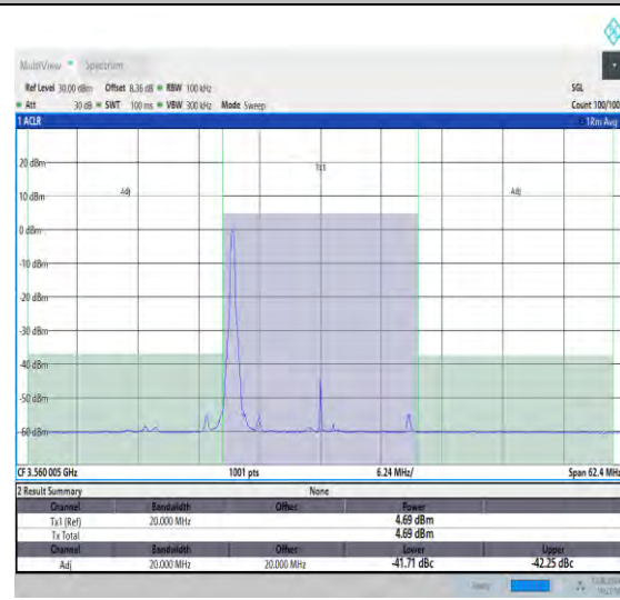
NTNV_N48_PC3_30_20_L_TID8_#1_-20_20
