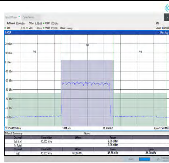
NTNV_N48_PC3_30_40_L_TID13_#1_-40_40
