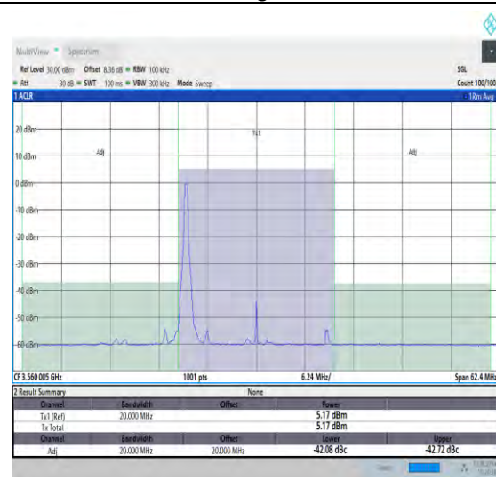
NTNV_N48_PC3_30_20_L_TID5_#1_-20_20
