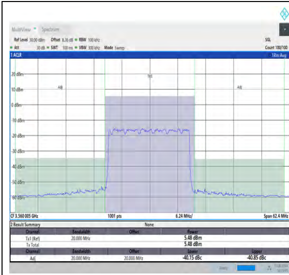
NTNV_N48_PC3_30_20_L_TID4_#1_+20_20
