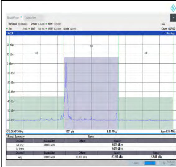
NTVN_N48_PC3_30_30_L_TID2_#1_+30_30
