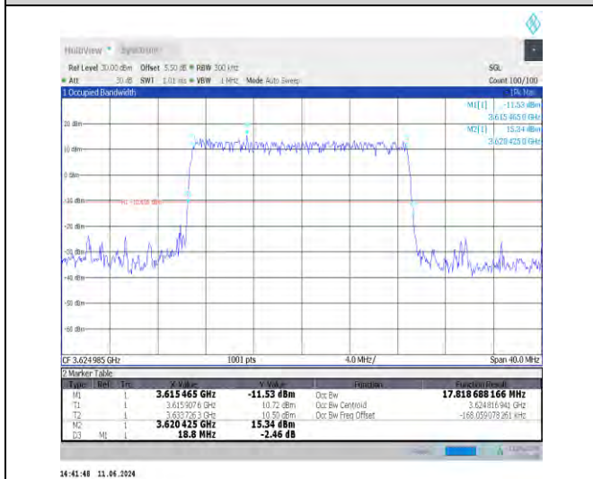
1-N48-30-20-M-2-DFT-PI2BPSK-Outer_Full-50@0-A nt0-17.819-18.800-≤20-PASS
