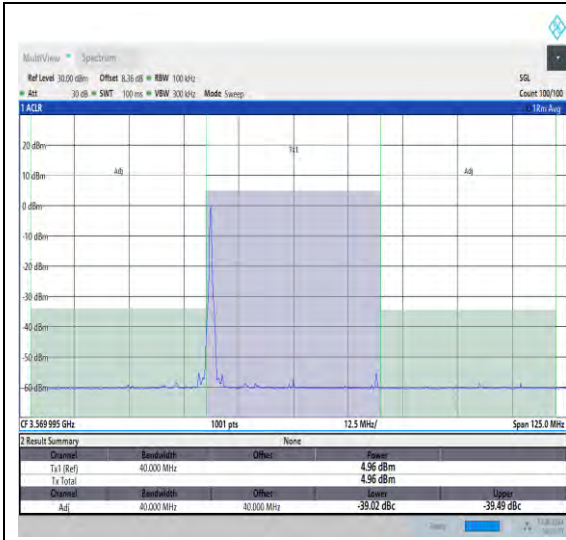
NTVN_N48_PC3_30_40_L_TID2_#1_-40_40
