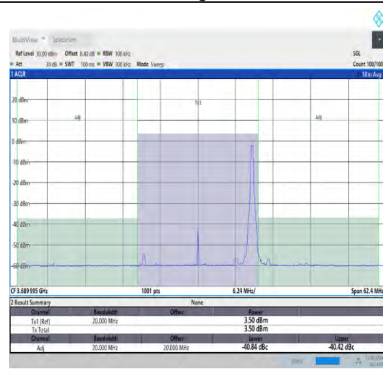
NTNV_N48_PC3_30_20_H_TID18_#1_-20_20
