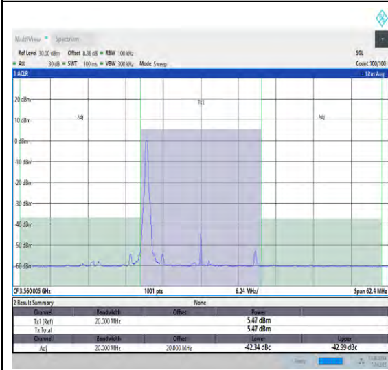
NTNV_N48_PC3_30_20_L_TID2_#1_+20_20
