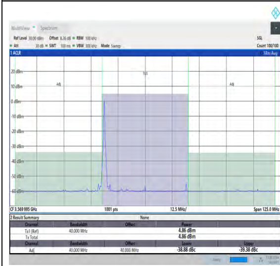
NTVN_N48_PC3_30_40_L_TID5_#1_-40_40
