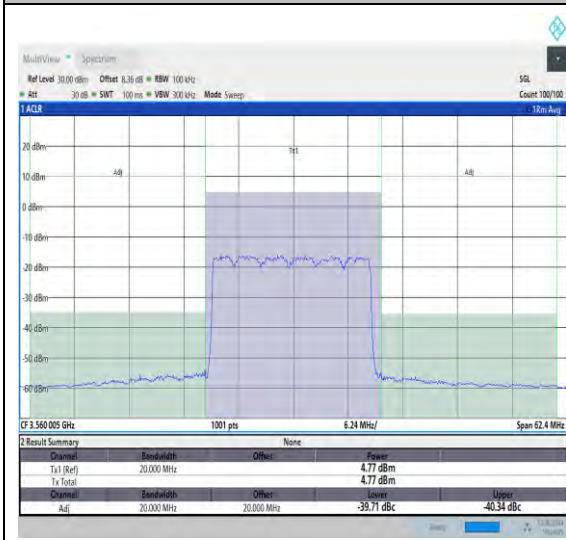
NTNV_N48_PC3_30_20_L_TID7_#1_-20_20
