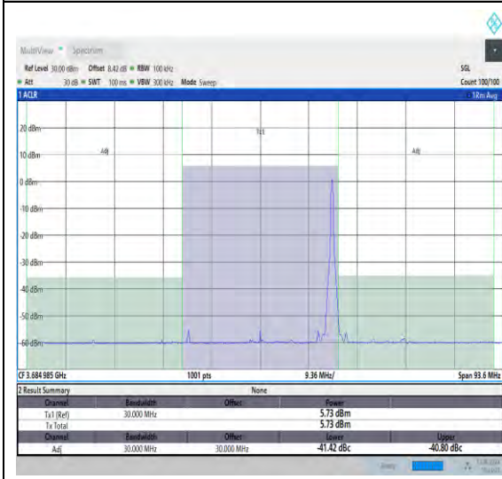
NTNV_N48_PC3_30_30_H_TID9_#1_30_30
