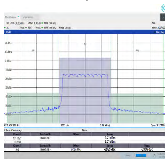
NTNV_N48_PC3_30_10_L_TID16_#1_-10_10
