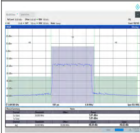
NTNV_N48_PC3_30_30_H_TID4_#1_-30_30
