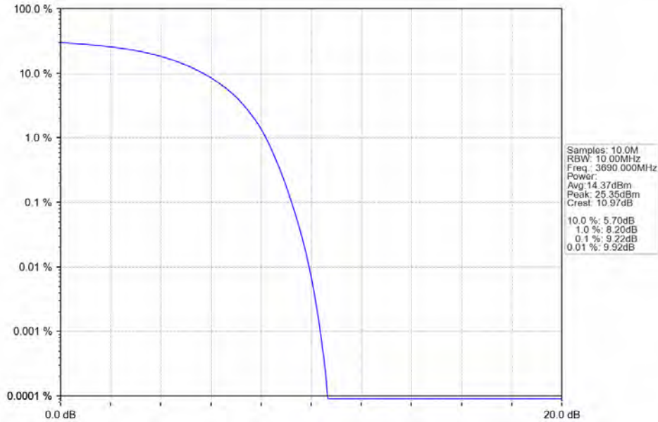
Band48_20MHz_QPSK_HCH_3690MHz_RB_100_0_NTNV
