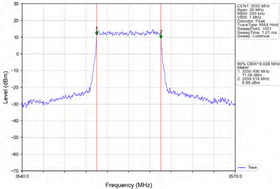
Band48_10MHz_QPSK_MCH_3625MHz_RB_50_0_NTNV
