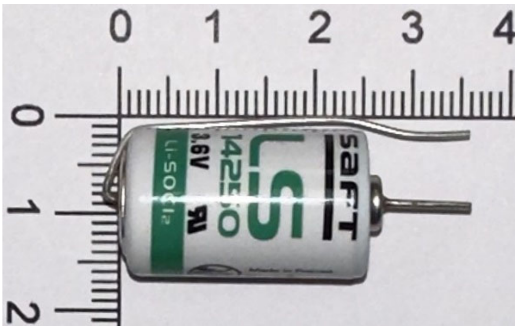
(3) EUT Photo
