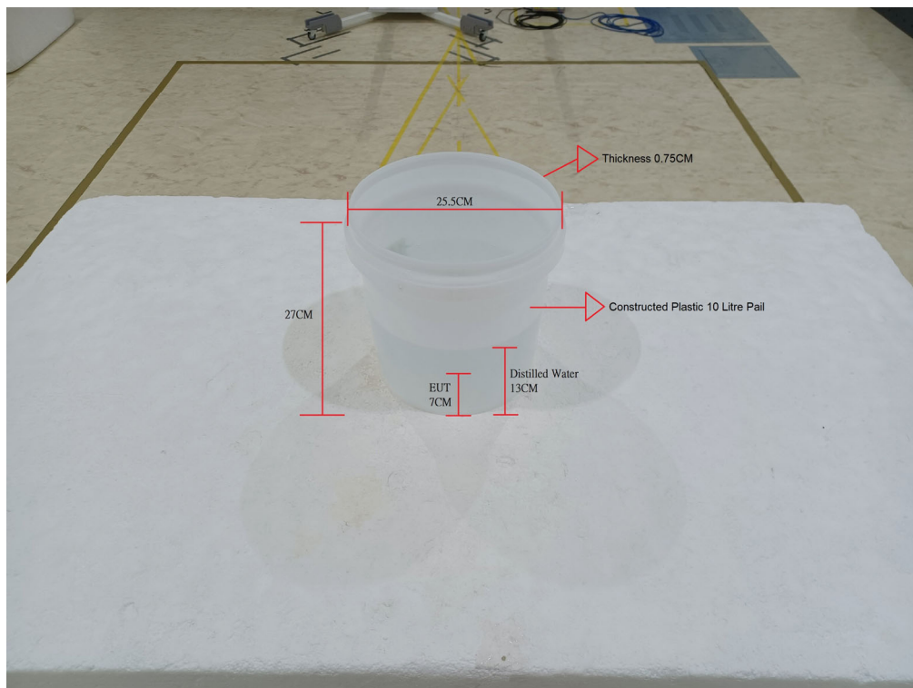
DUT Position
