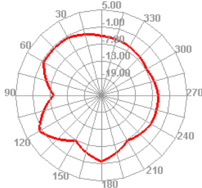
5650.000MHz H
