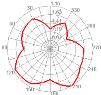
5650.000MHz E1
