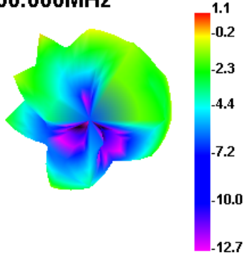
5650.000MHz E1
