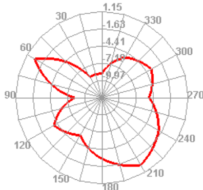
5650.000MHz E2
