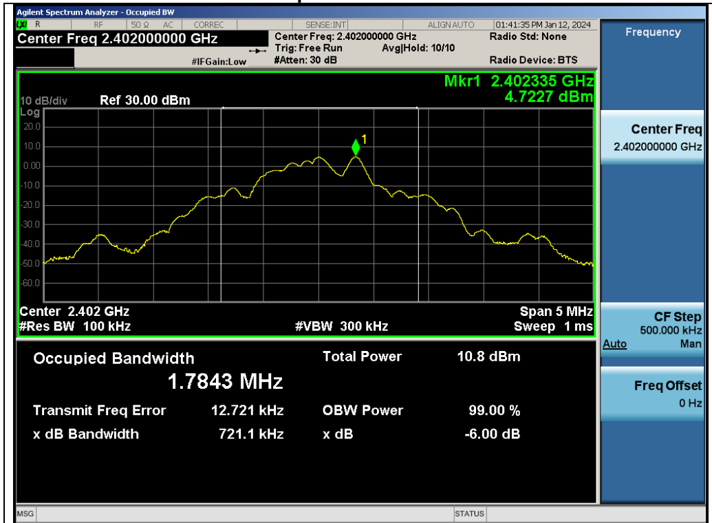
Test_Graph_GFSK_ANT1_2402_DTSBW
