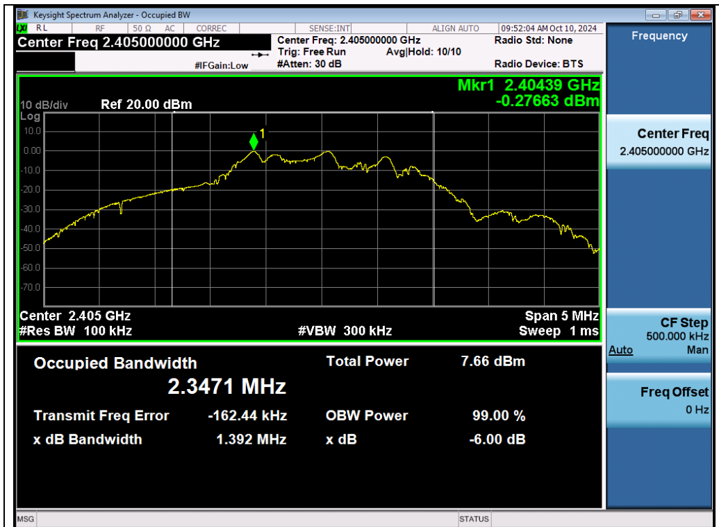
Test_Graph_2.4G_ANT1_2405_DTBSBW
