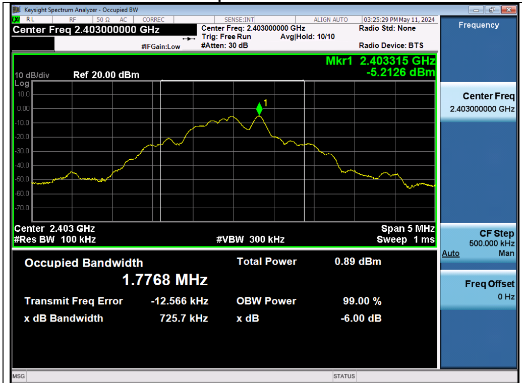
Test_Graph_GFSK_ANT1_2403_DTSBW
