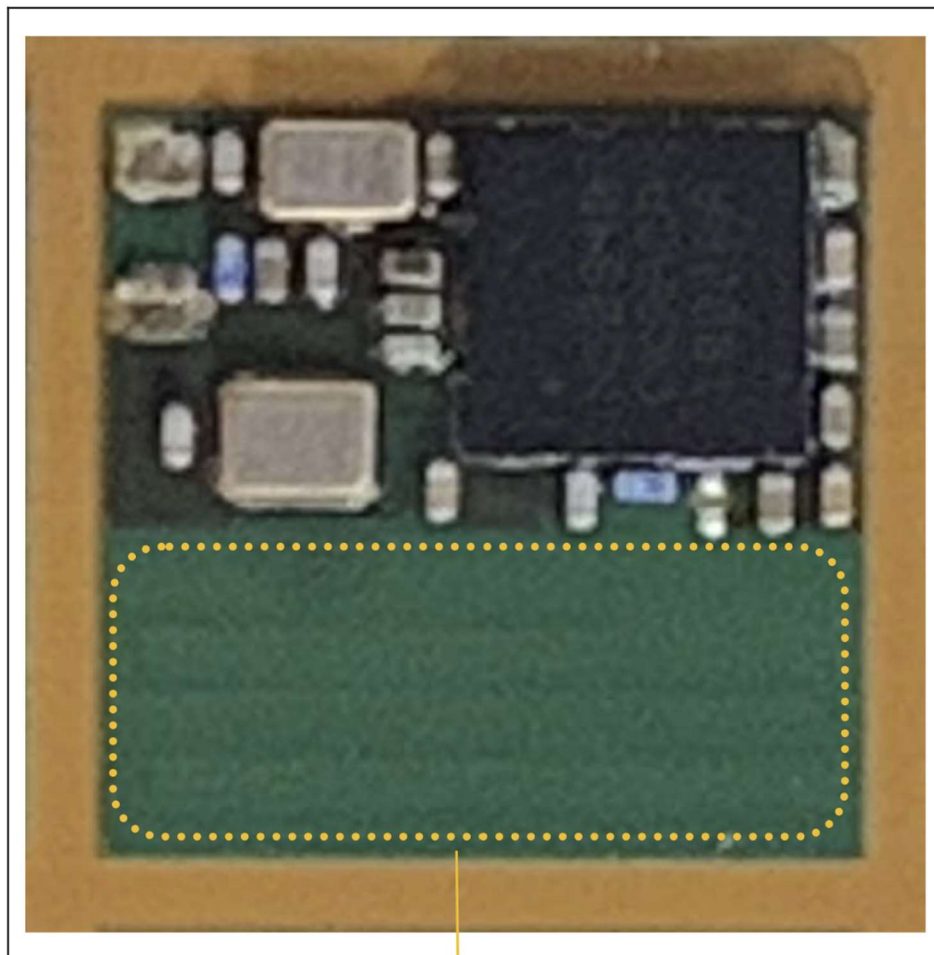
Antenna Area
