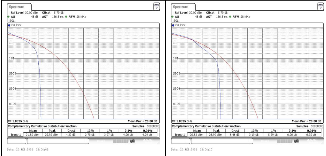
Band25-1.4MHz-QPSK-26365-1RB#0-PASS Band25-1.4MHz-16QAM-26365-1RB#0-PASS
