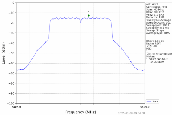
802.11ax(HEW20) HCH 5825MHz SU / Ant1 NTN
