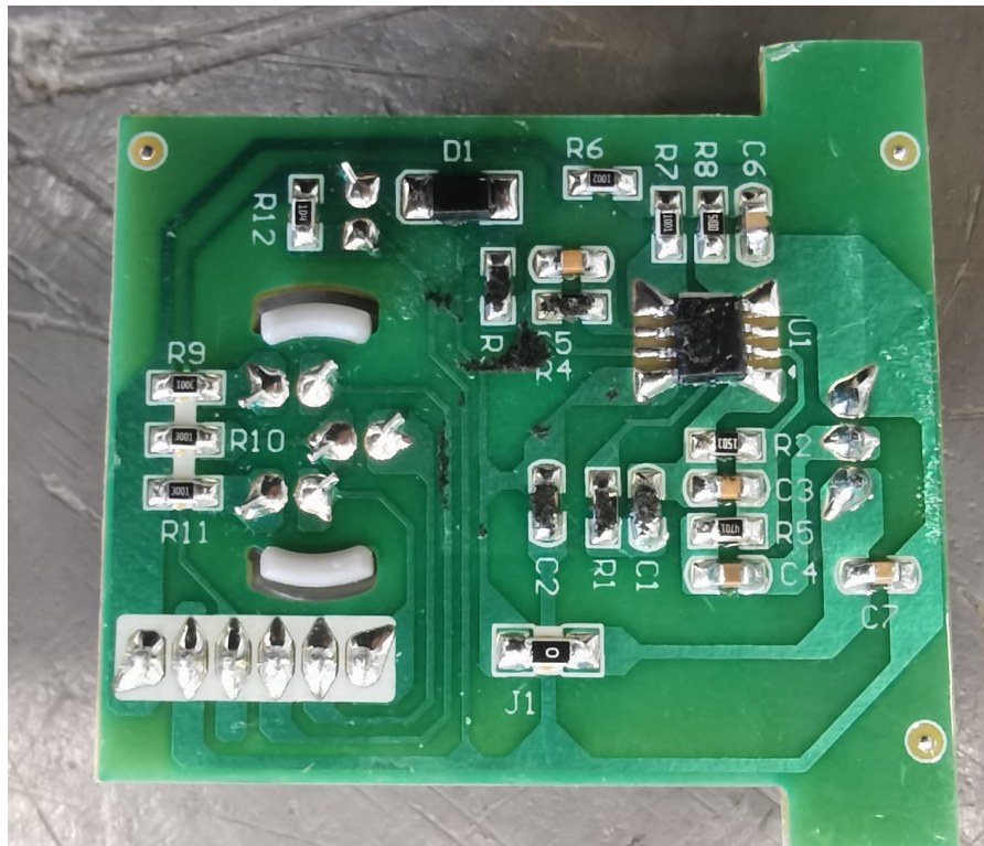
Photo 18– 24GHz RF Module
