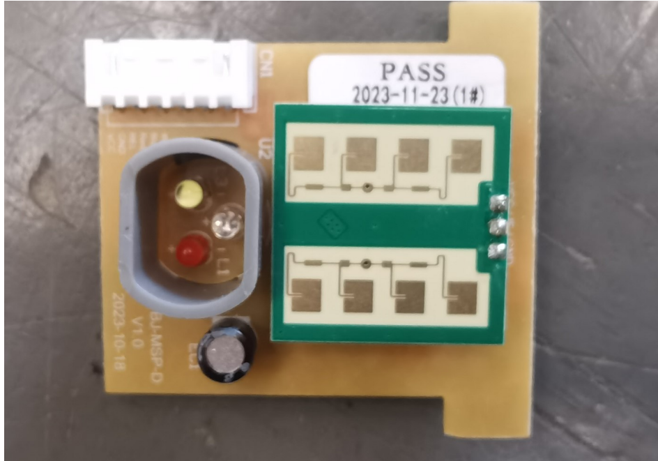
Photo 17– 24GHz RF Module
