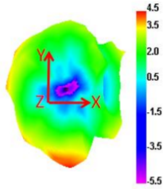
E1 Face 5240MHz
