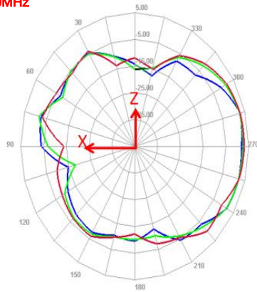
E1 Face 5240MHz
