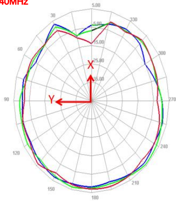
Horizontal 5240MHz
