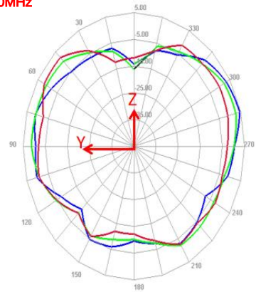
E2 Face 5240MHz
